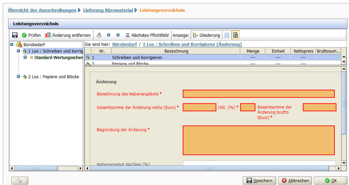
Abbildung 7.38: Änderung im Leistungsverzeichnis für Nebenangebot ohne Hauptangebot erfassen
