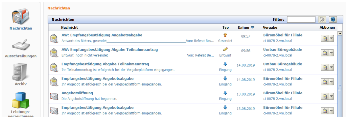
Abbildung 6.21: Bereich Nachrichten
