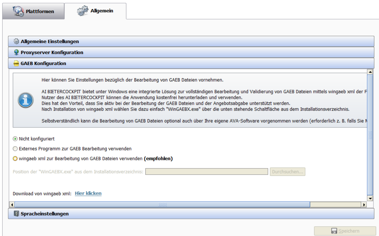
Abbildung 6.10: GAEB Konfiguration
