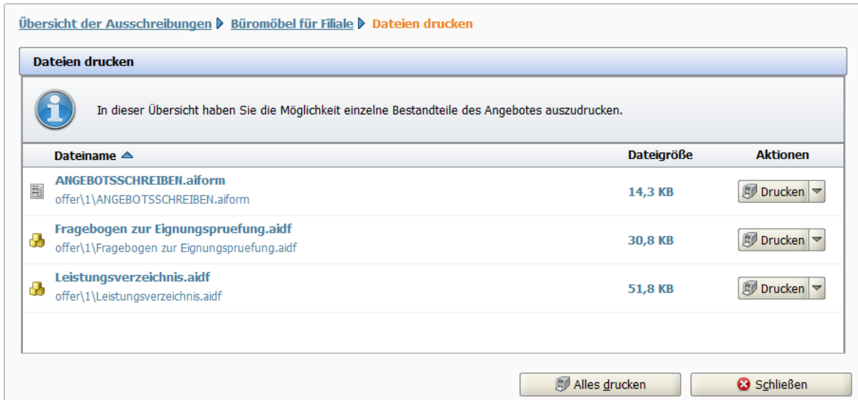
Abbildung 7.75: Angebot drucken
