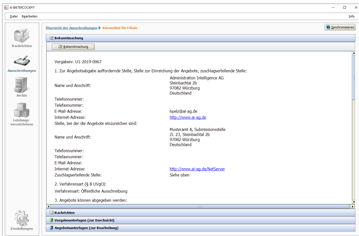
Abbildung 7.2: Ausschreibungen - Bekanntmachung
