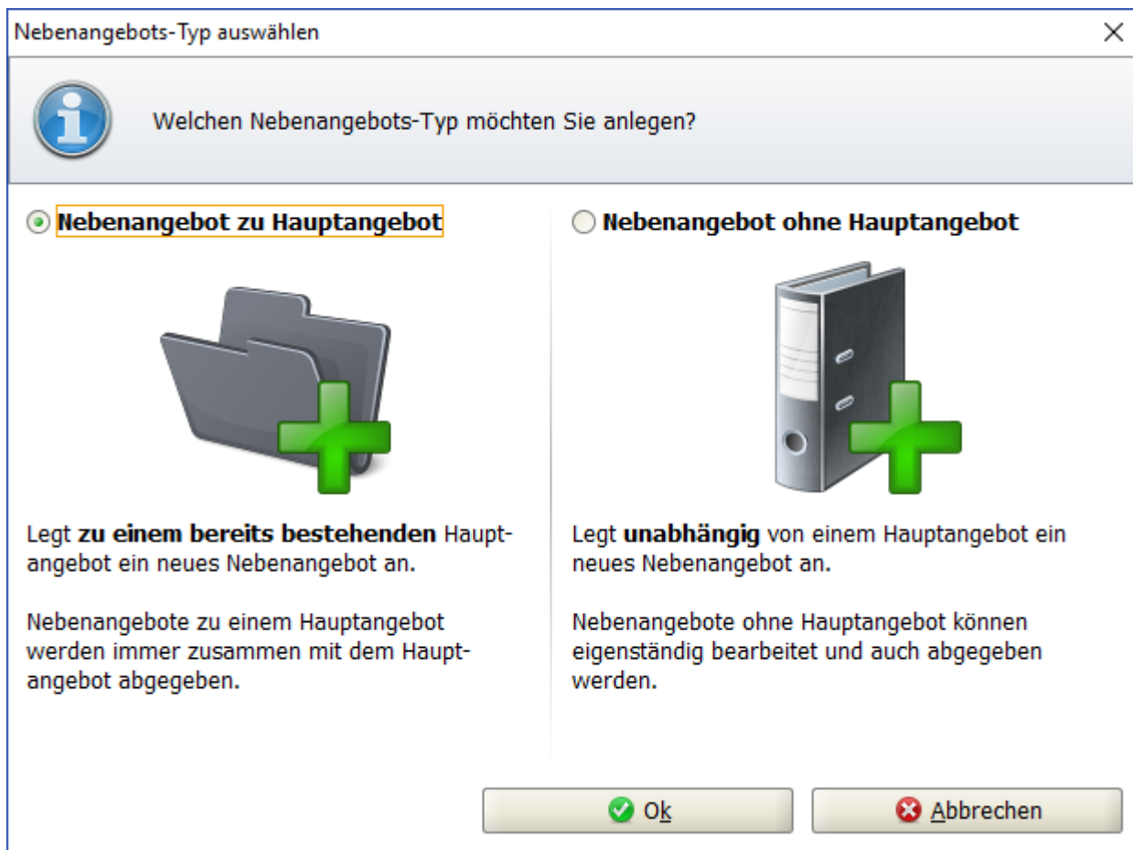
Abbildung 7.31: Nebenangebotstyp wählen
