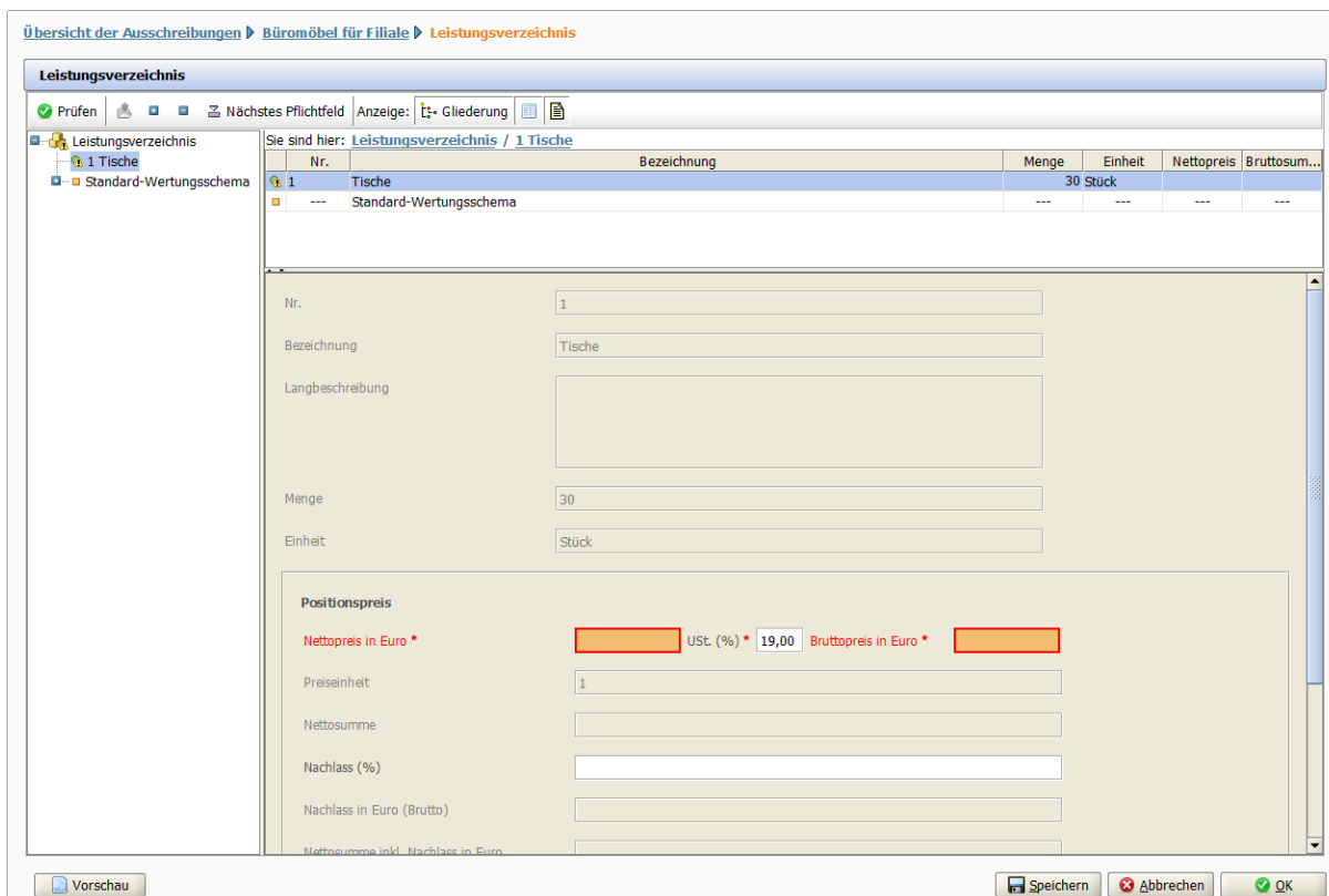
Abbildung 7.16: Leistungsverzeichnis
