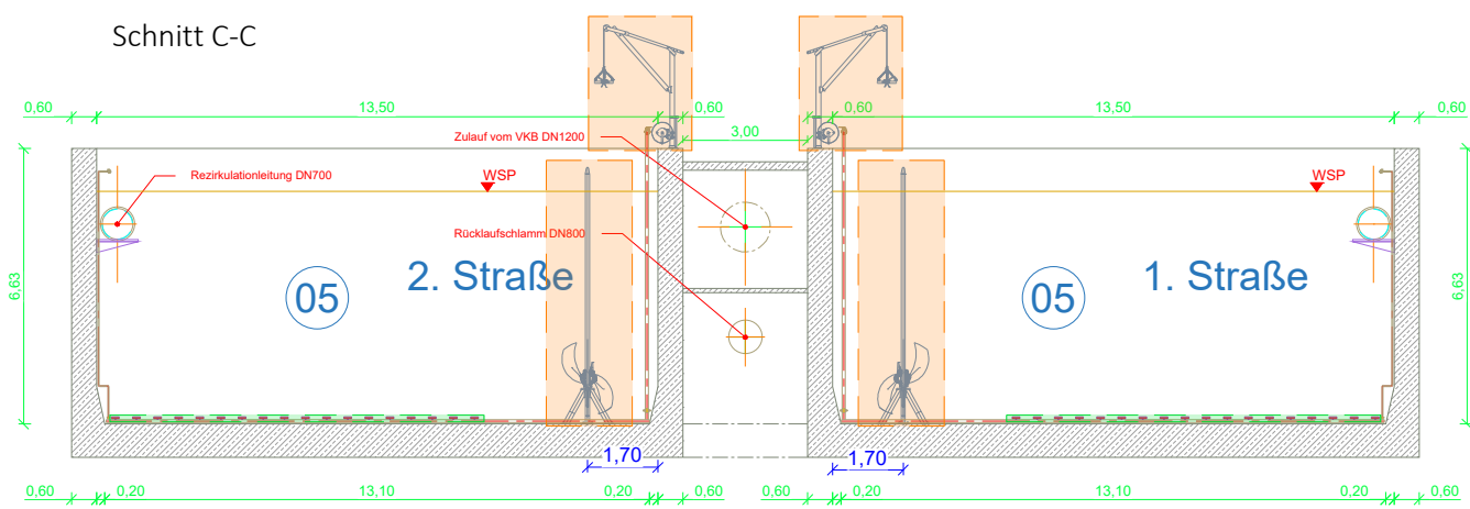
Schnitt C-C
