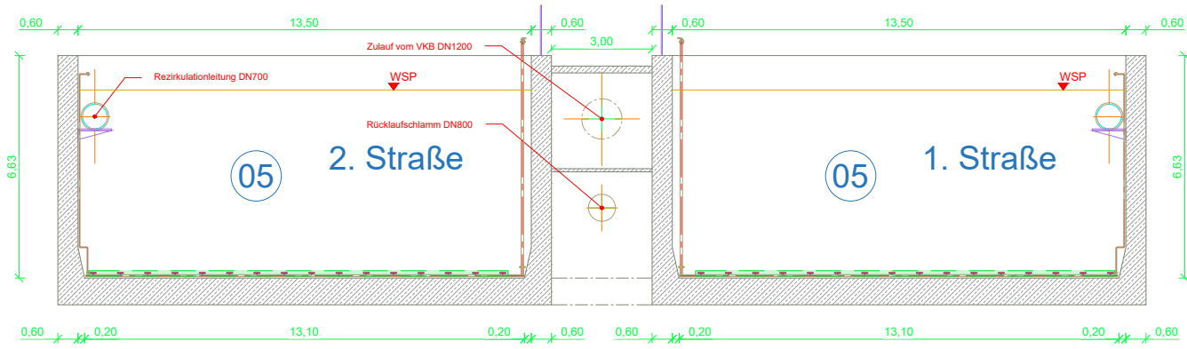
Schnitt C-C
