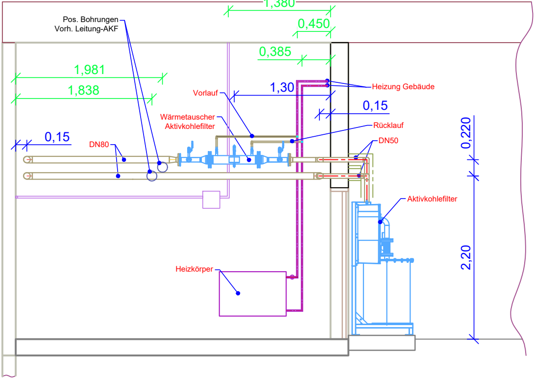
Links (Innen) Schnitt B-B
