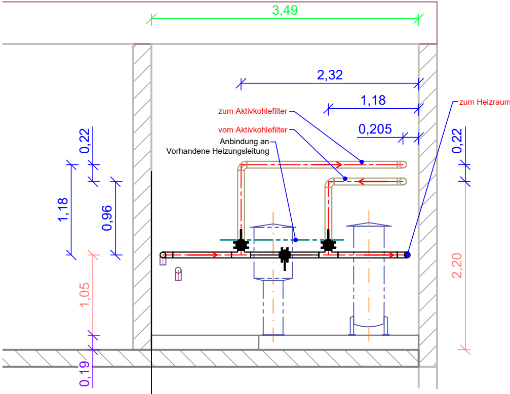
Vorne Schnitt A-A
