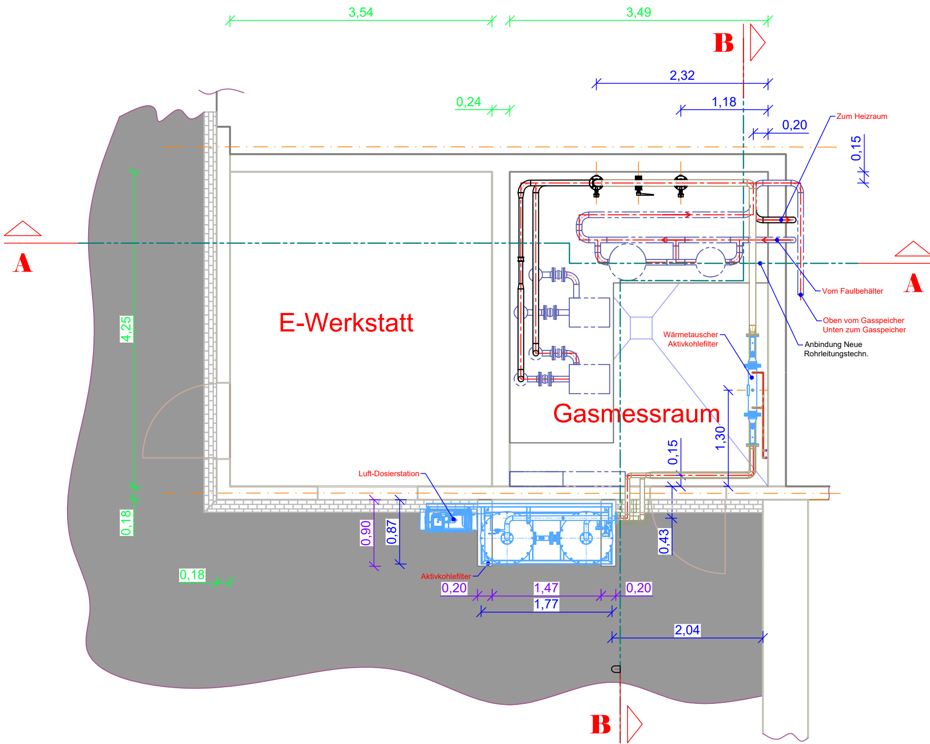
Draufsicht
