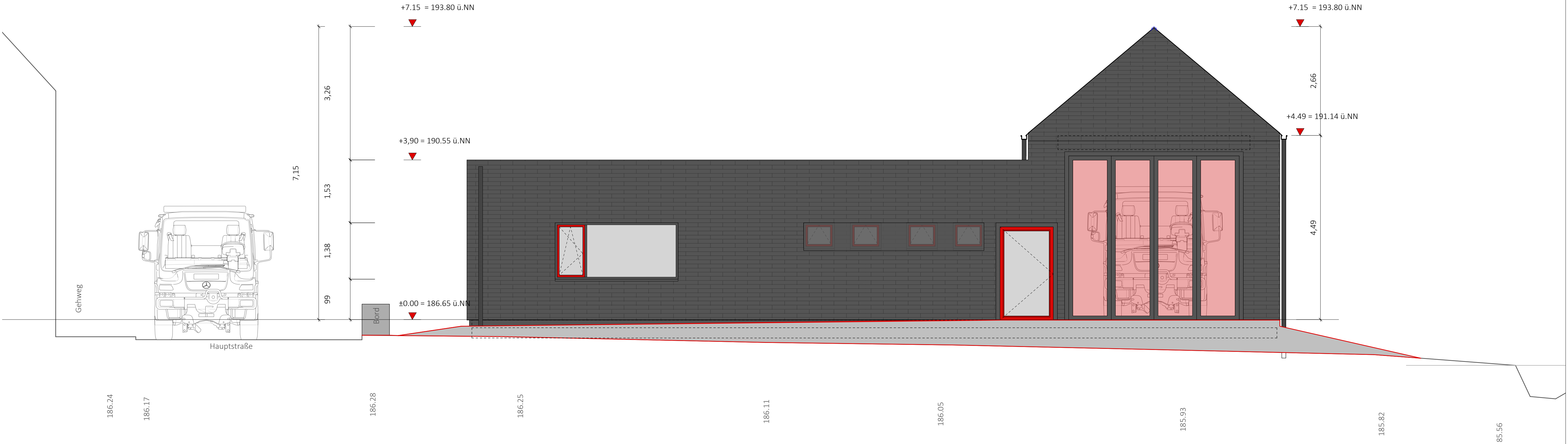
Ansicht Nord
