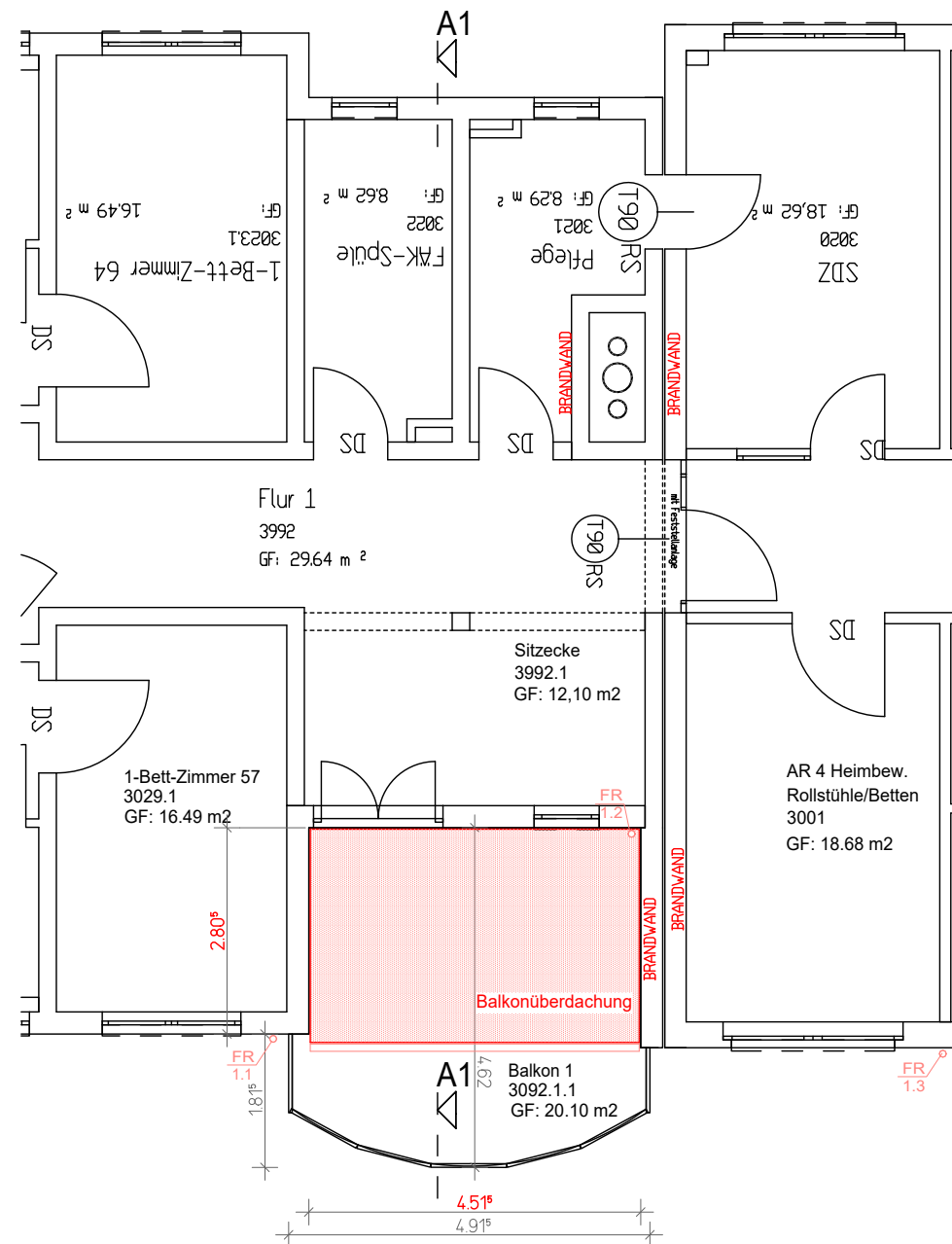
GRUNDRISS 2.OG HAUS 1B - Block A1
