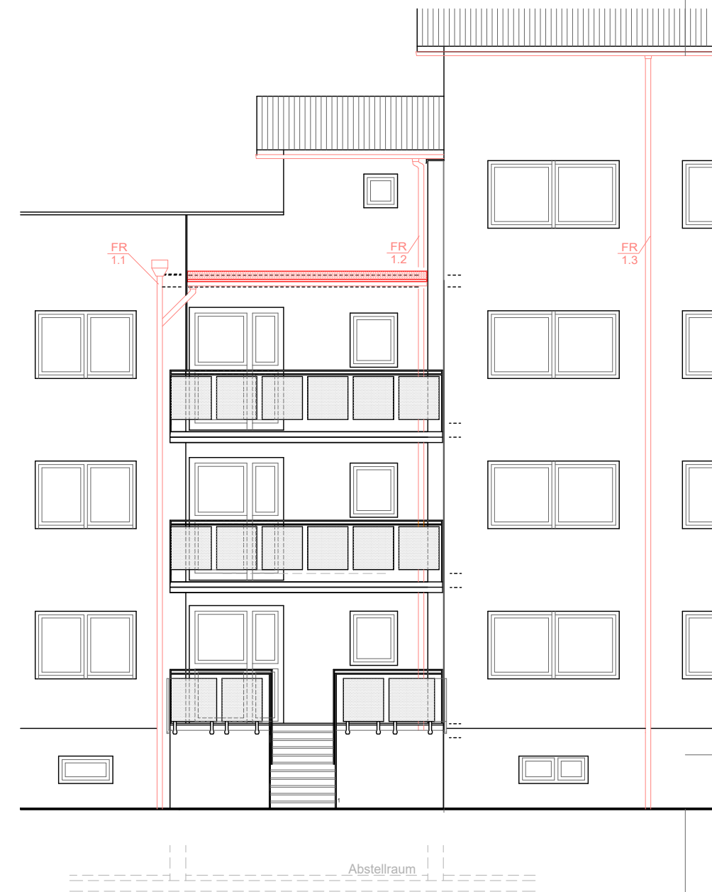
OSTANSICHT HAUS 1B Block A1
