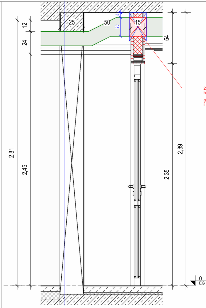
Schnitt Pos. 08 M 1 : 20
