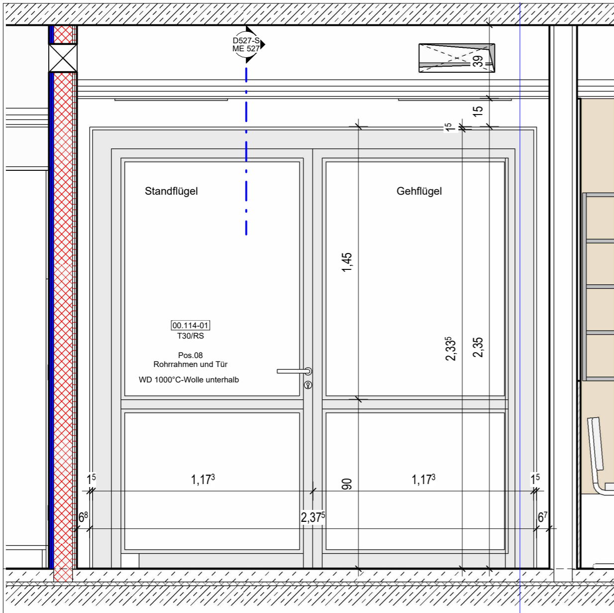
Ansicht Pos. 08 M 1 : 20
