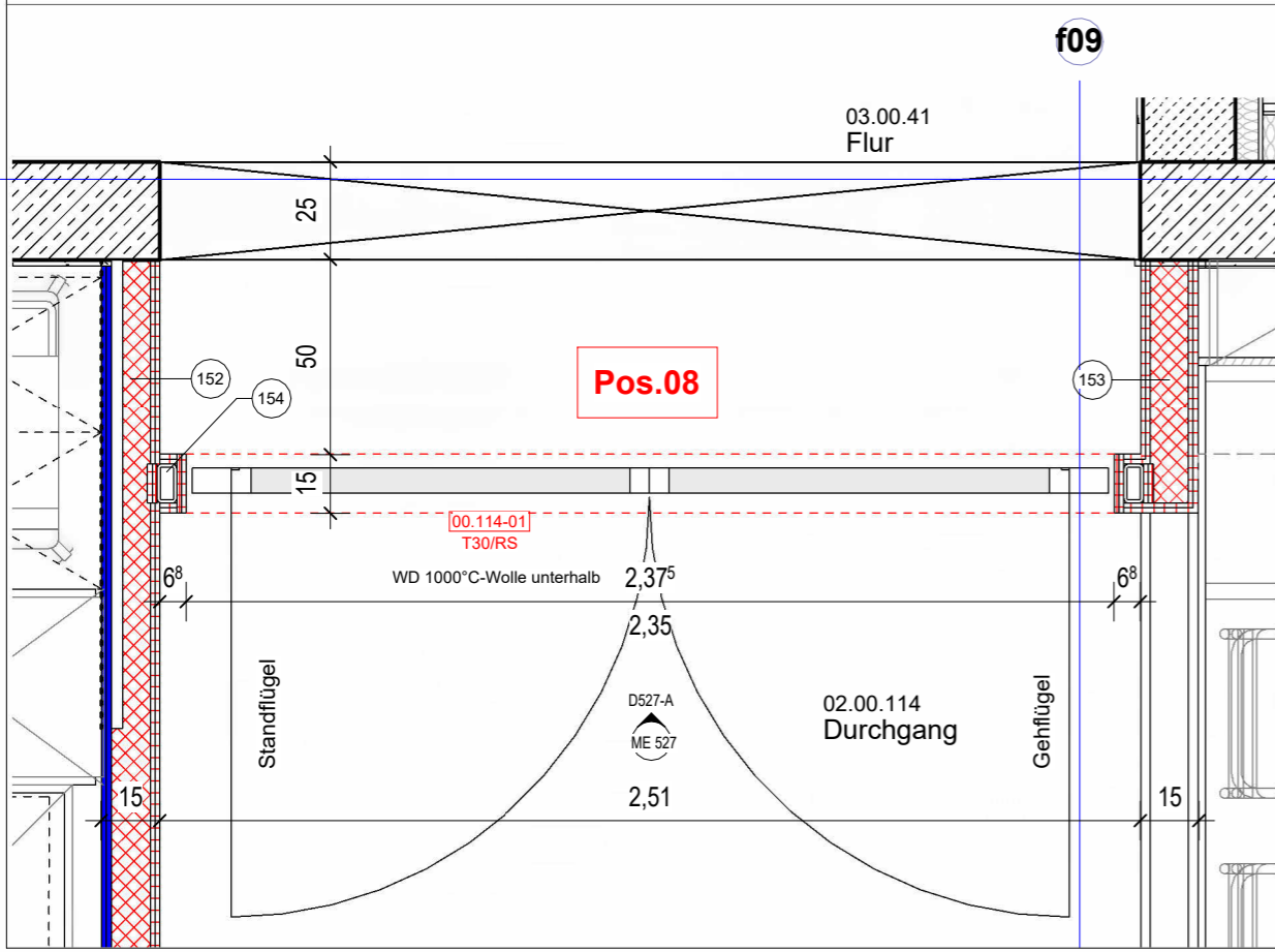
Grundriss Pos.08 M 1 : 20
