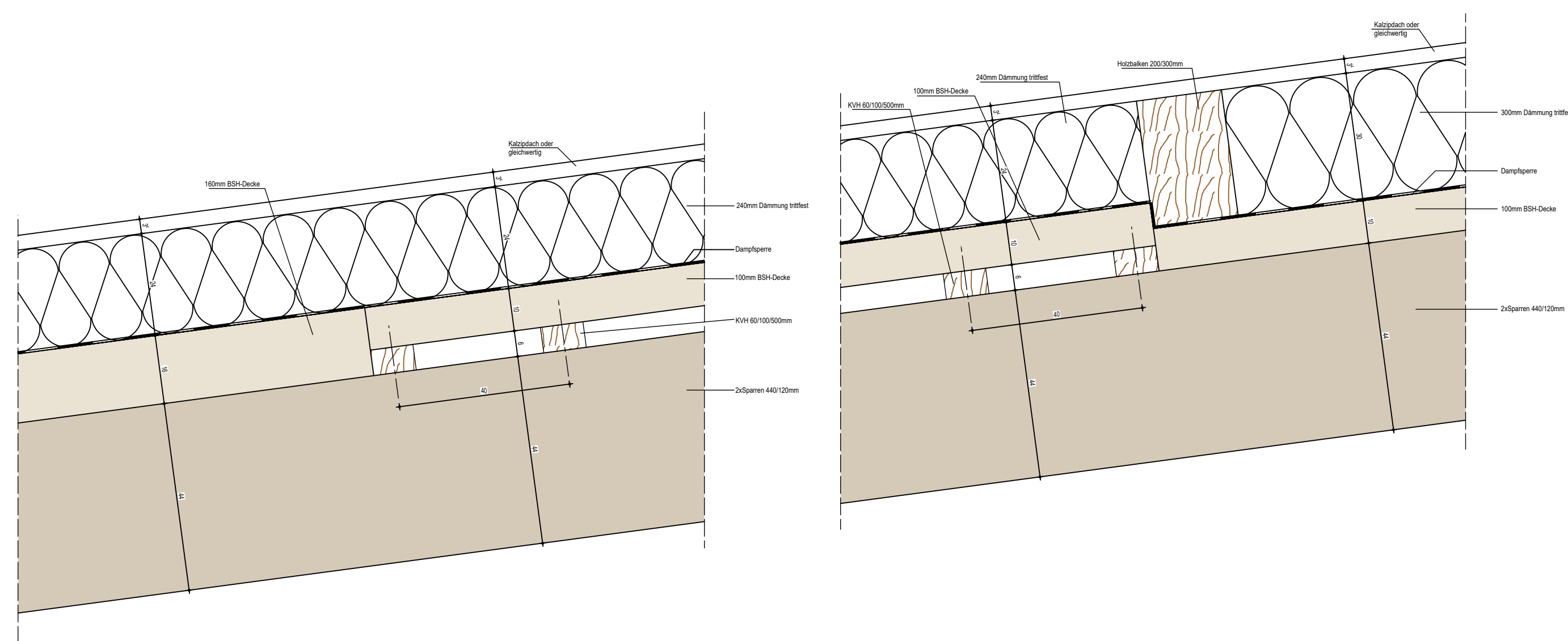
Detail Dachaufbauten M 1:10
