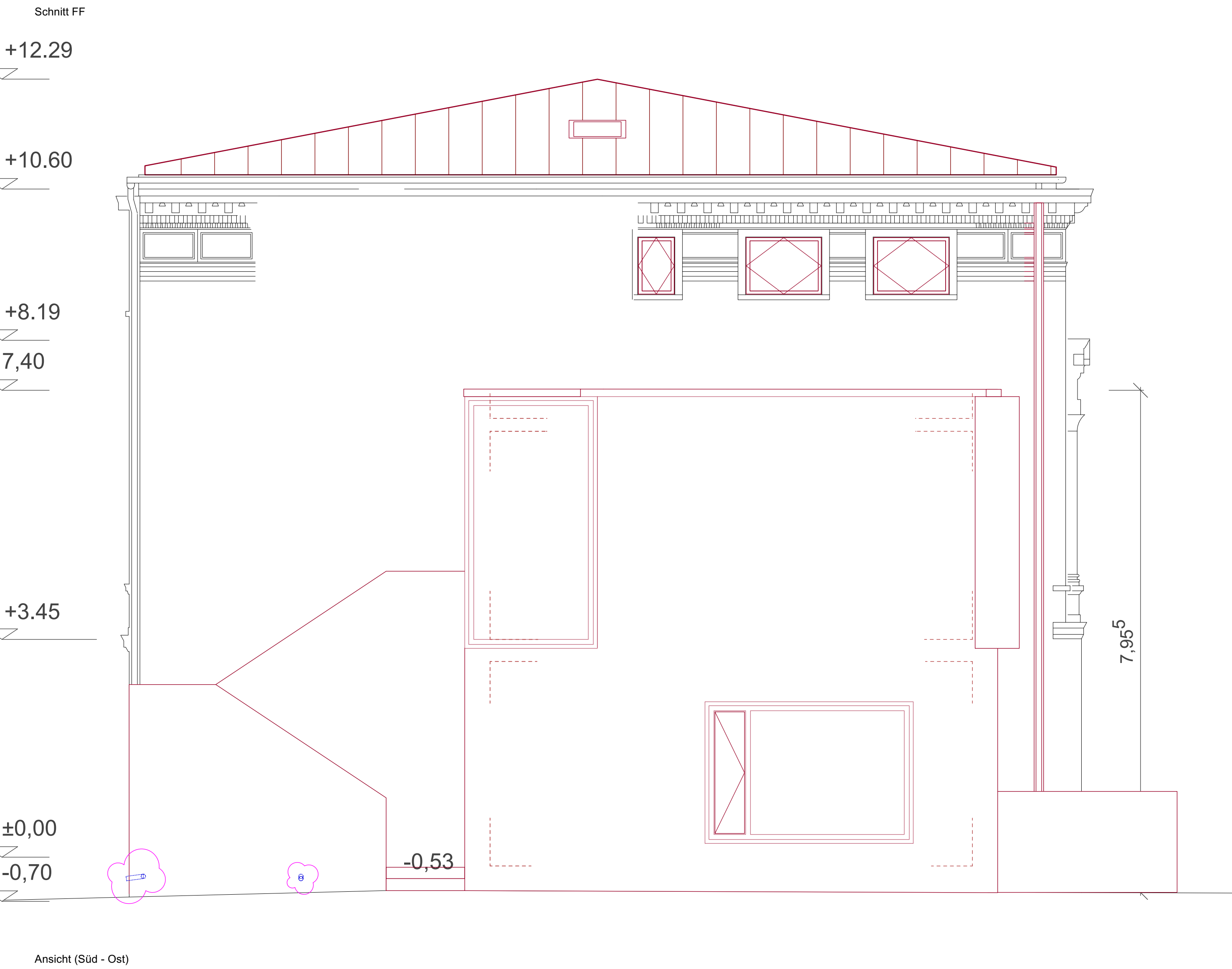
Ansicht (Süd - Ost)
