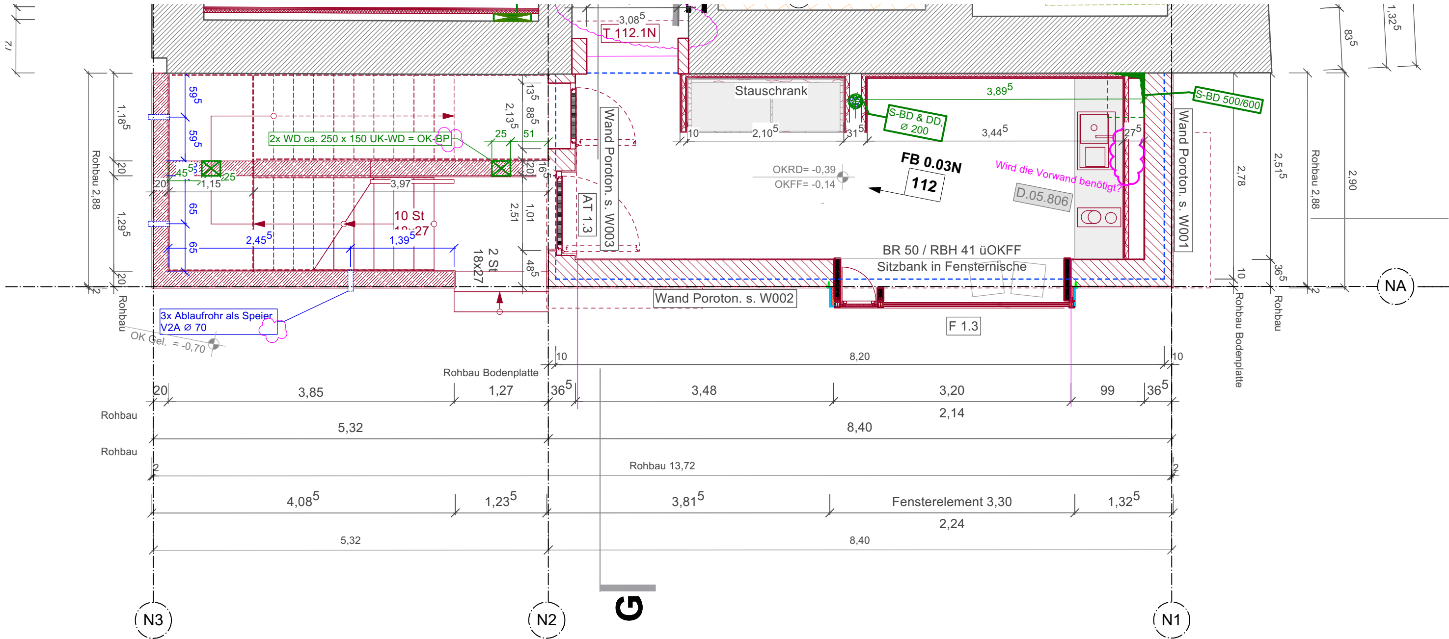
Grundriss EG
