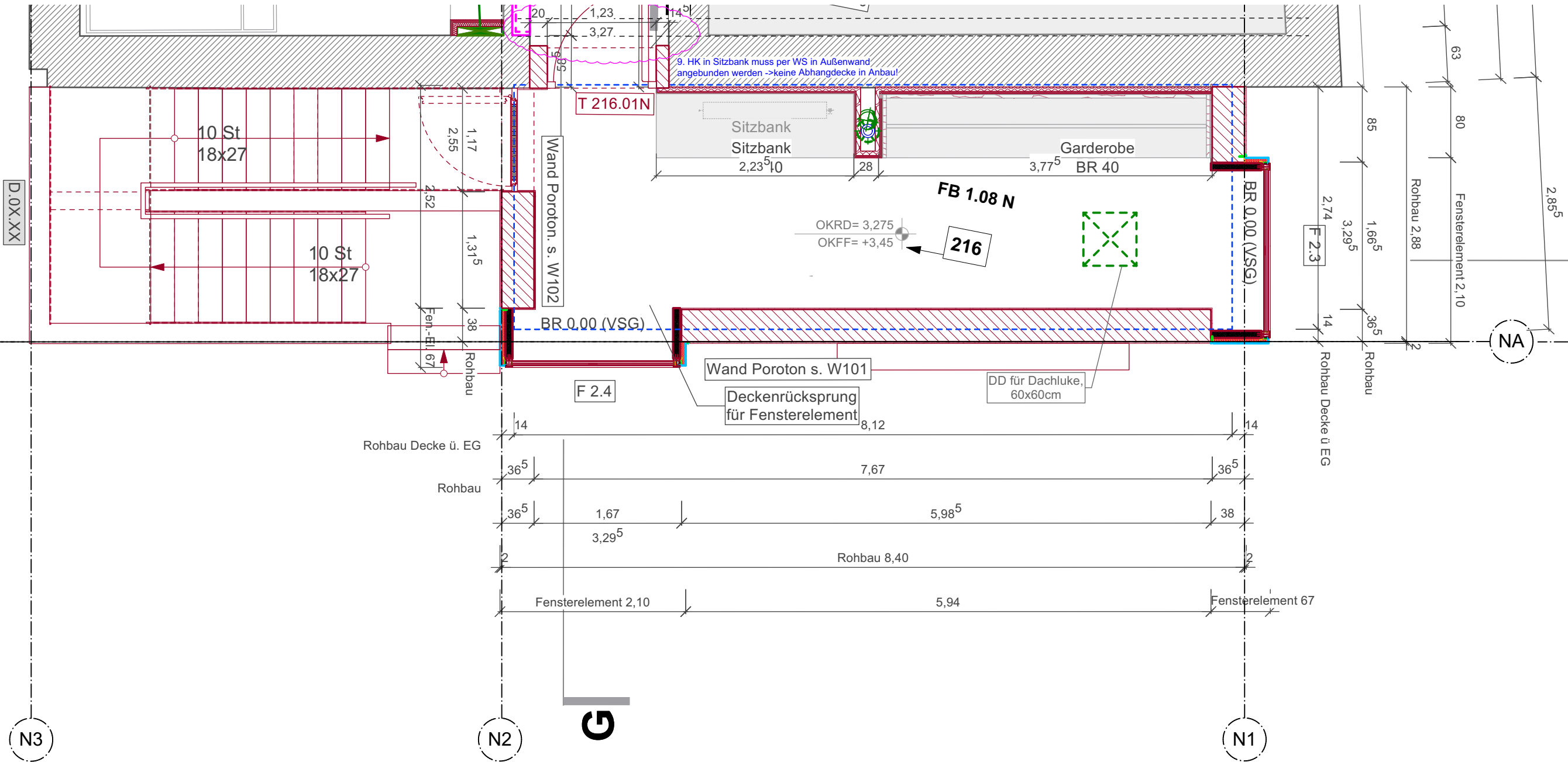
Grundriss OG
