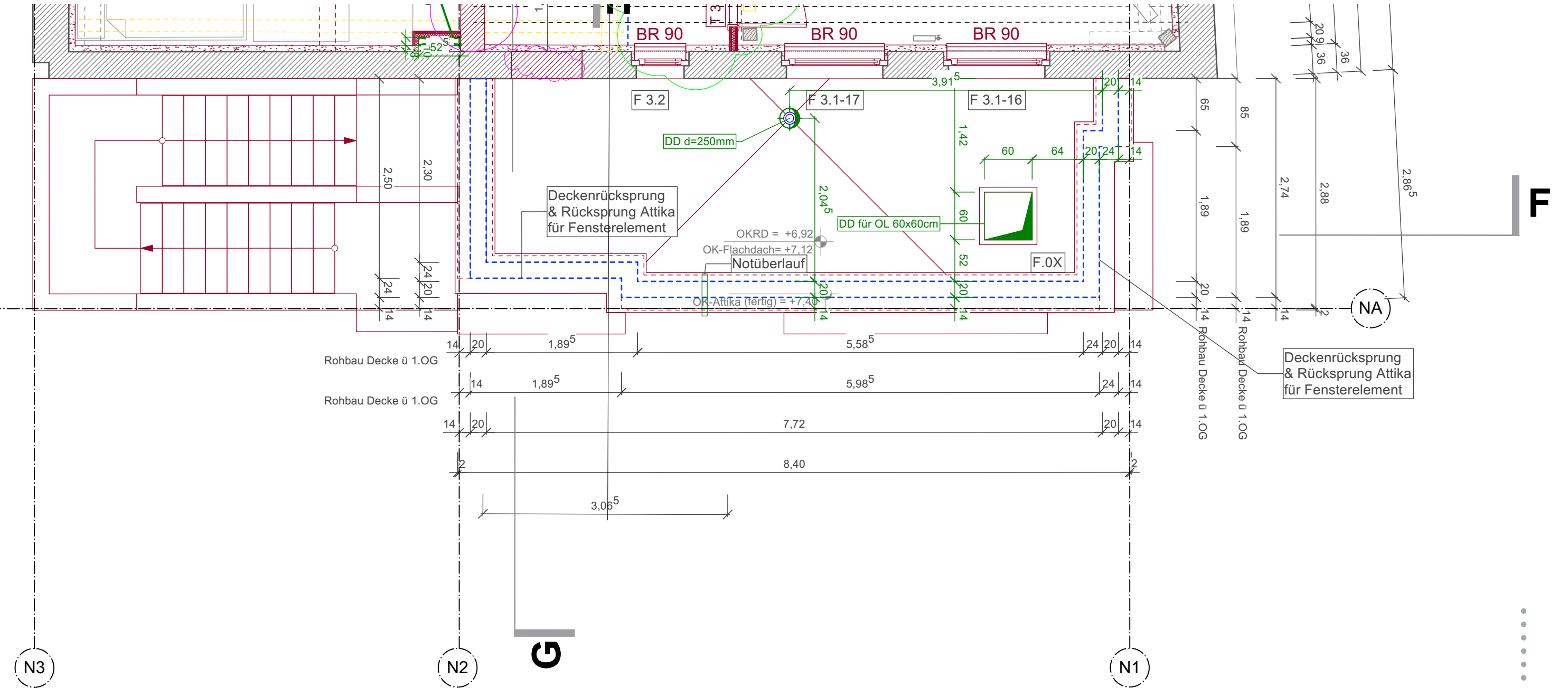
Grundriss DG
