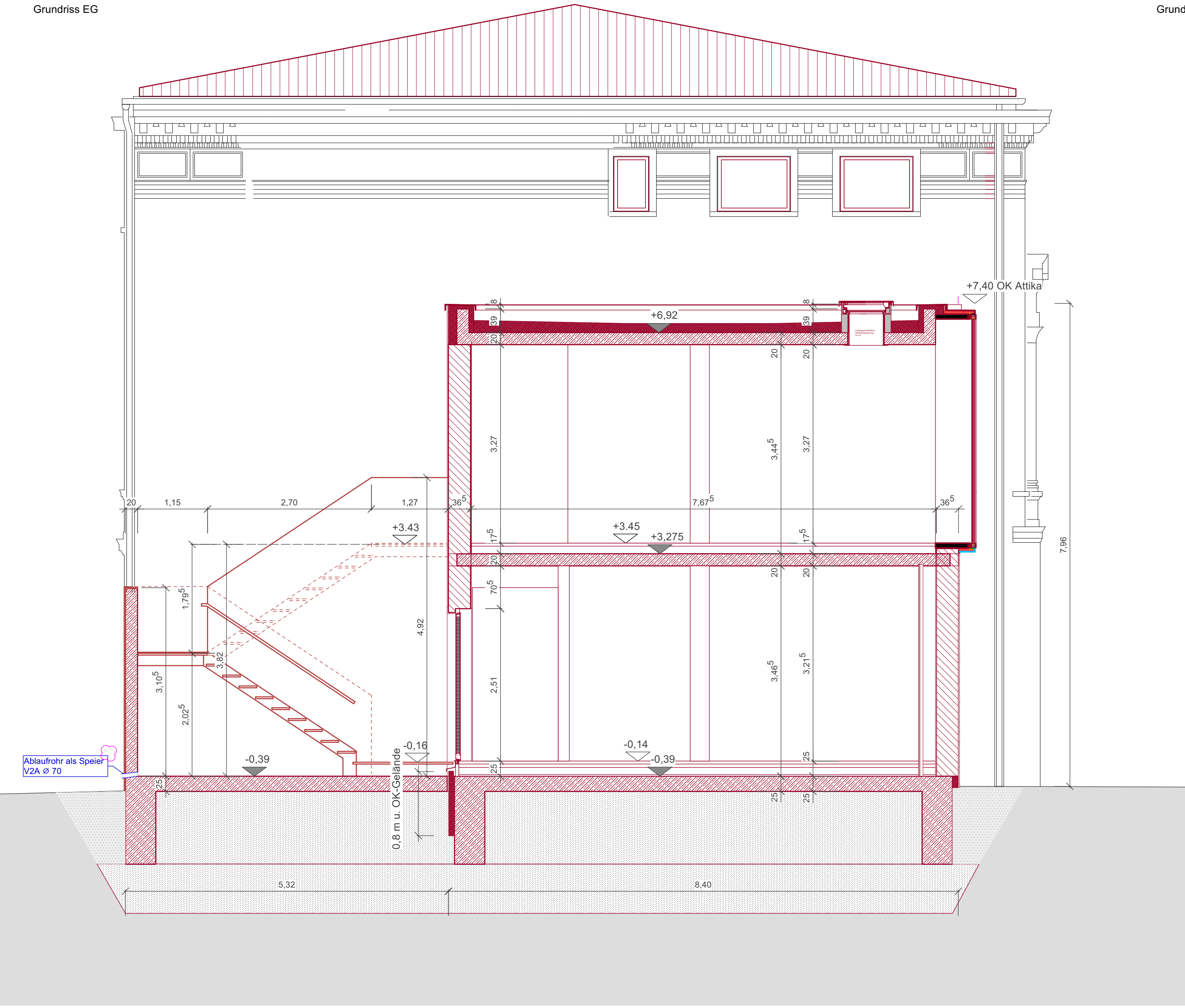
Schnitt FF
