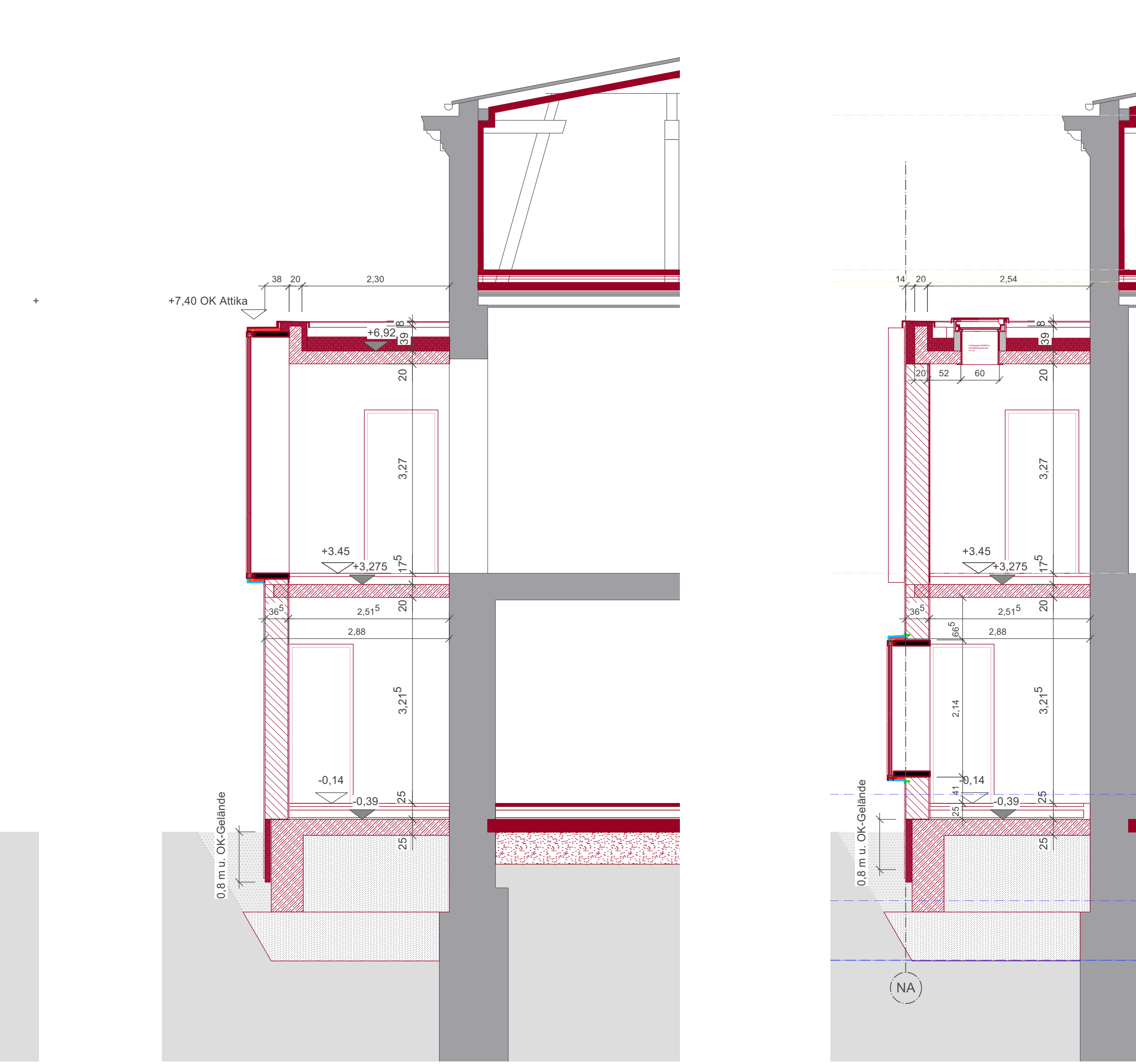
Schnitt GG
