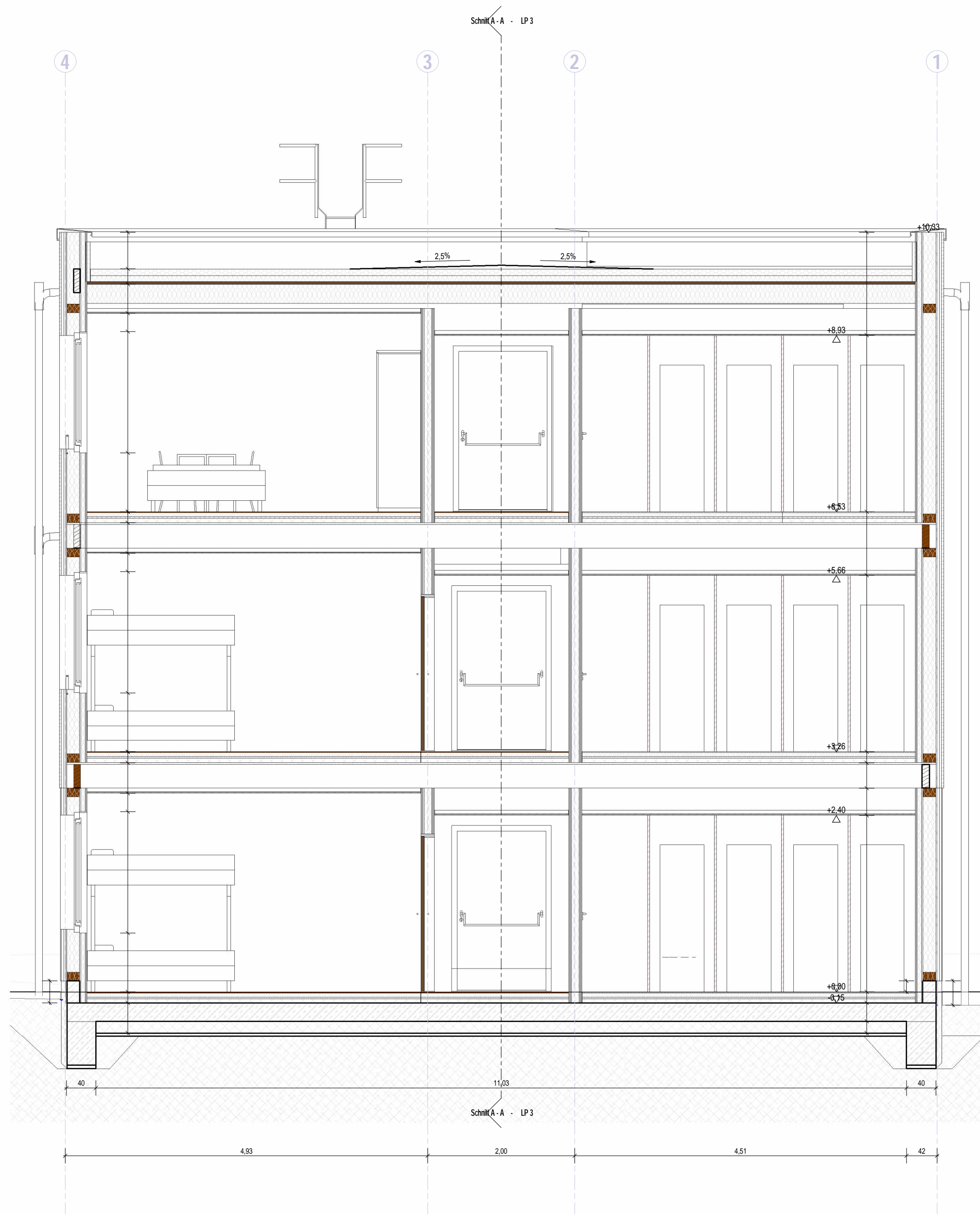
Schnitt B - B - LP 3 M 1:50
