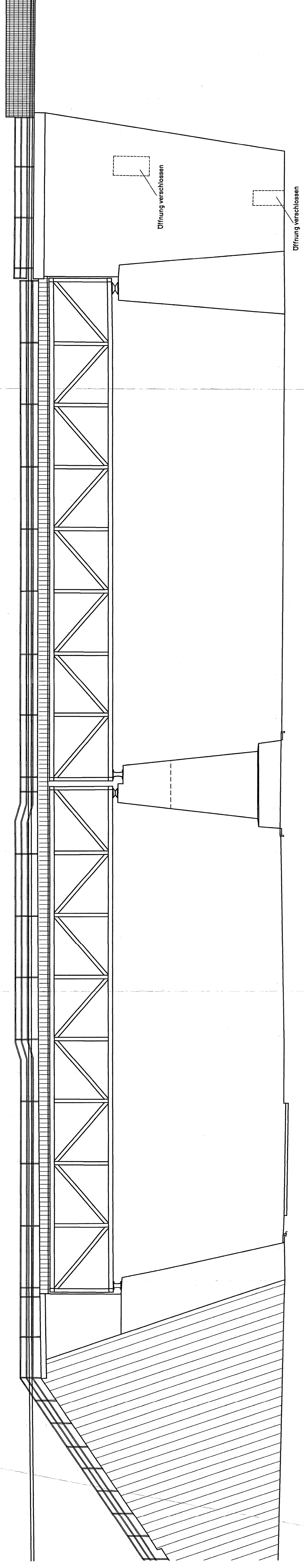
Ansicht von Osten M. 1:100
