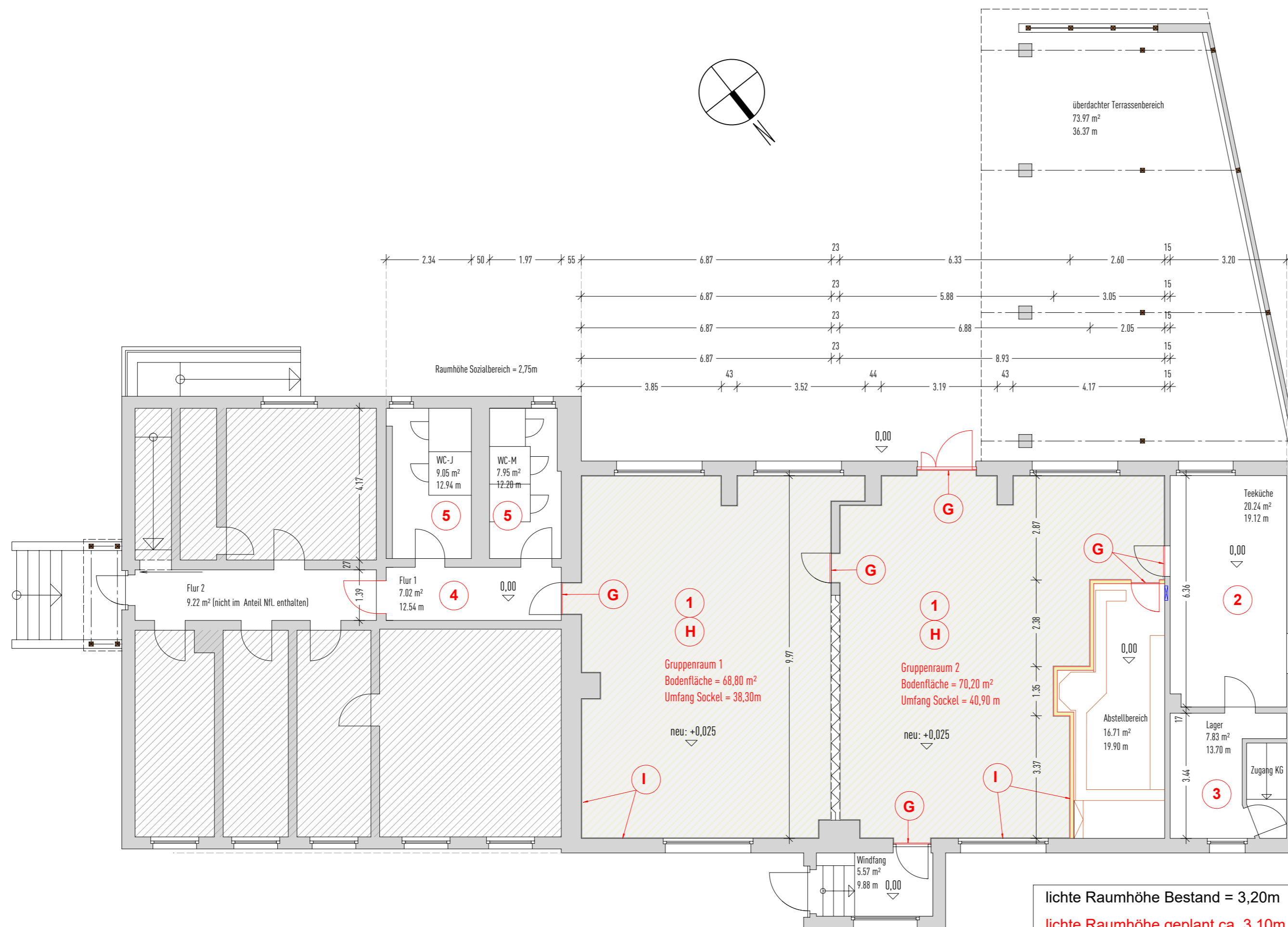
Grundriss Erdgeschoss Sportlerheim Baalberge - neu als Ersatzunterkunft für den Hort Baalberge
