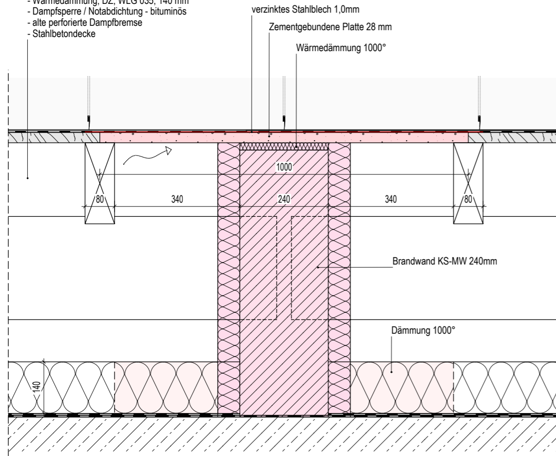
QUERSCHNITT BRANDWAND - BEREICH zw. ACHSE 3-4
