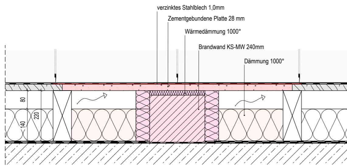
QUERSCHNITT BRANDWAND - BEREICH zw. ACHSE 3-4
