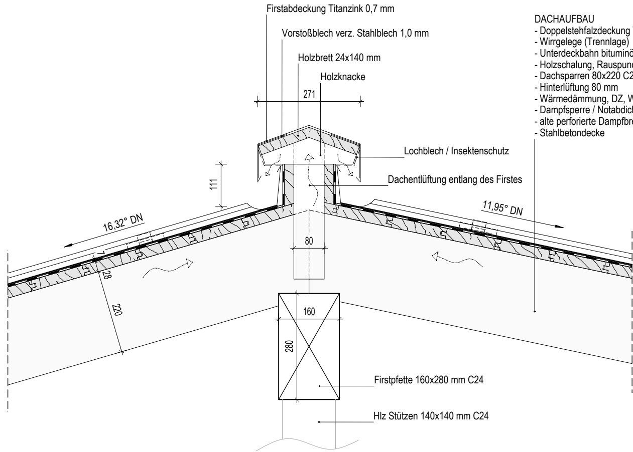
FIRSTANSCHLUSS
