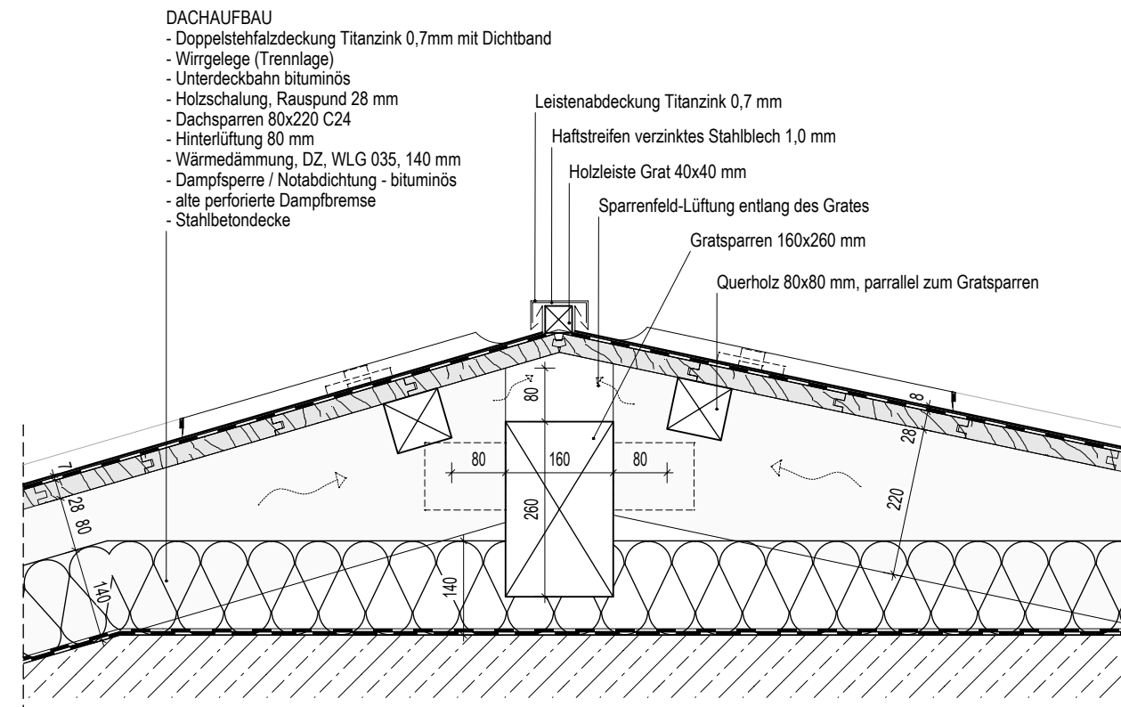
GRATANSCHLUSS
