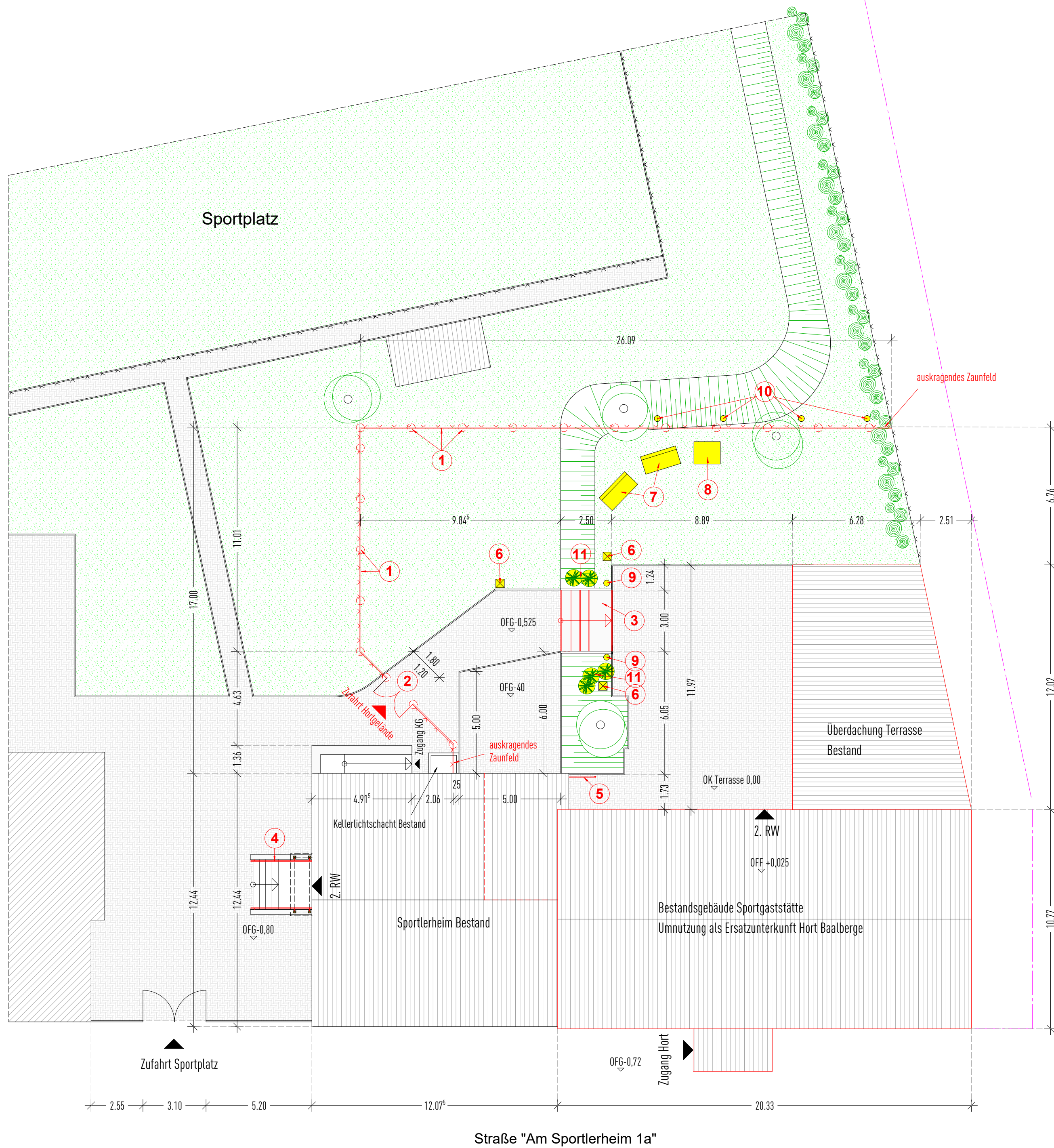
Lageplan Außenanlagen - 1:200
