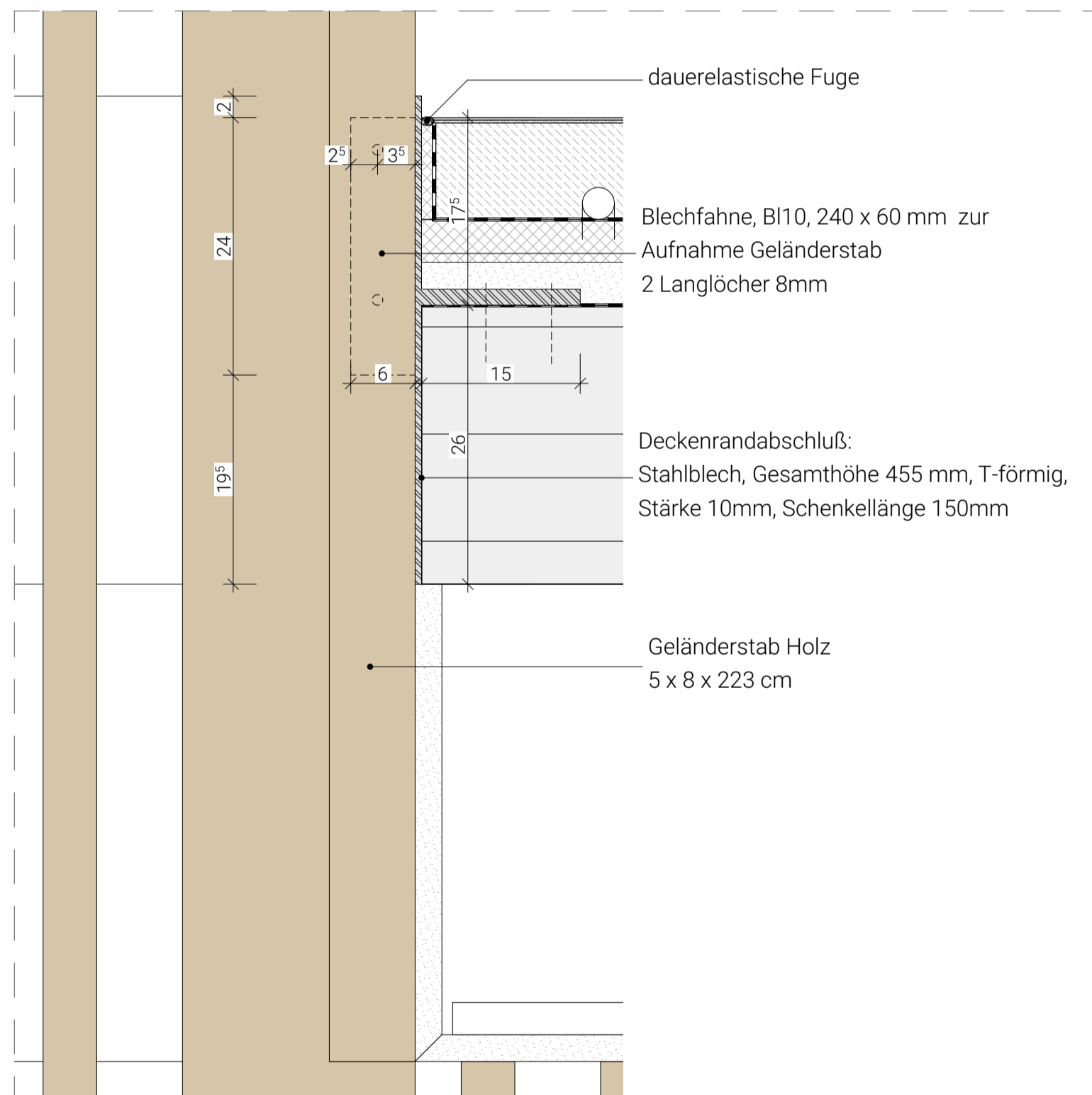
Innengeländer Deckenrand M1:5
