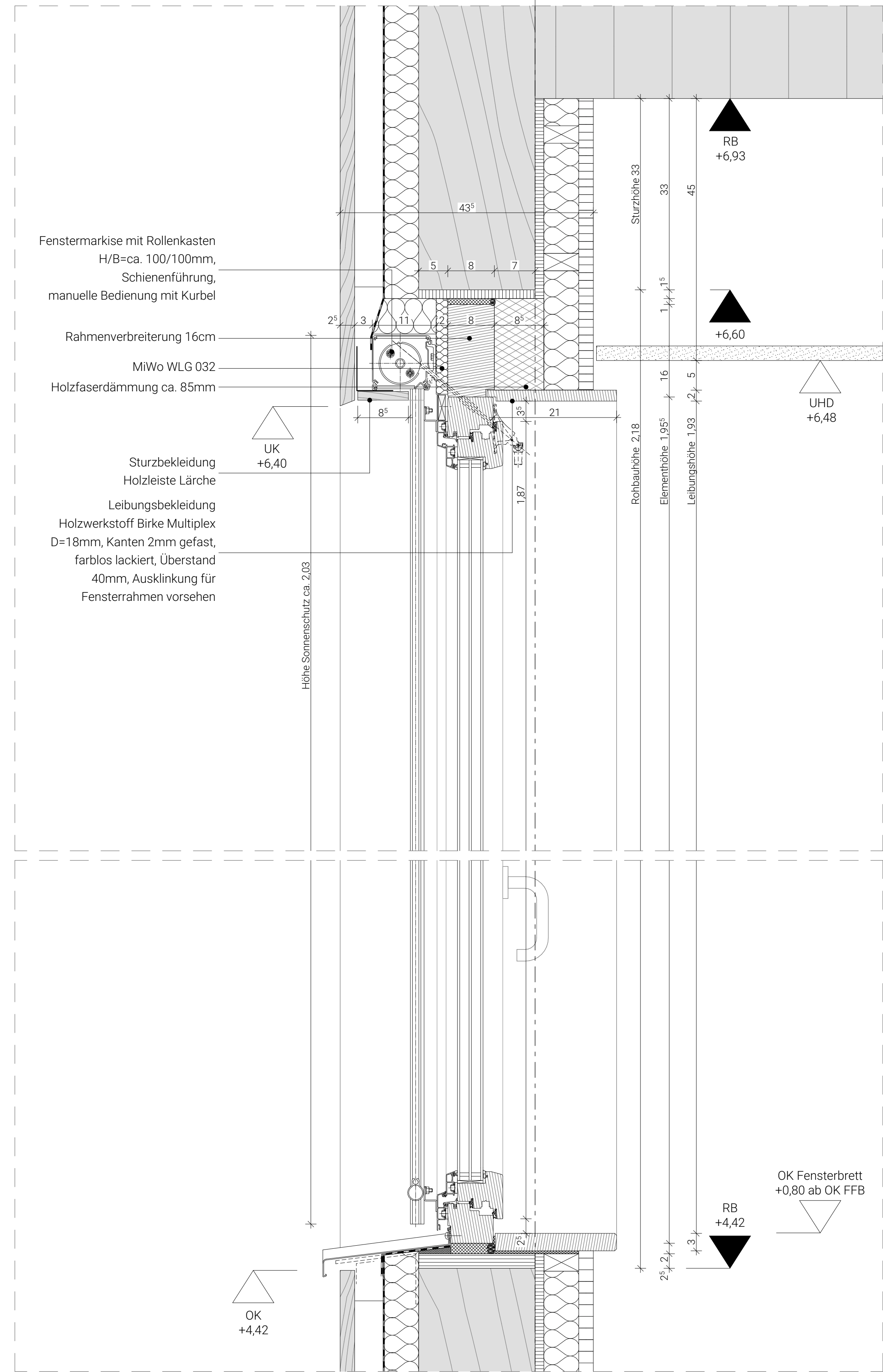
Schnitt BB' M 1:5
