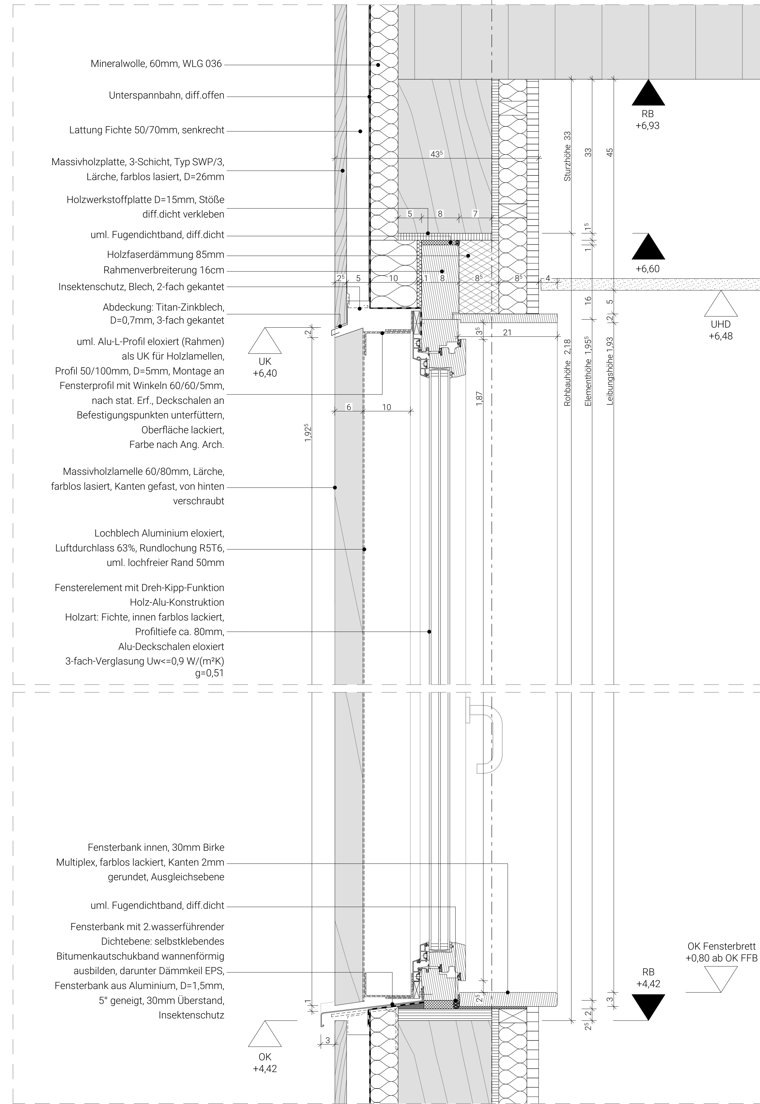
Schnitt AA' M 1:5
