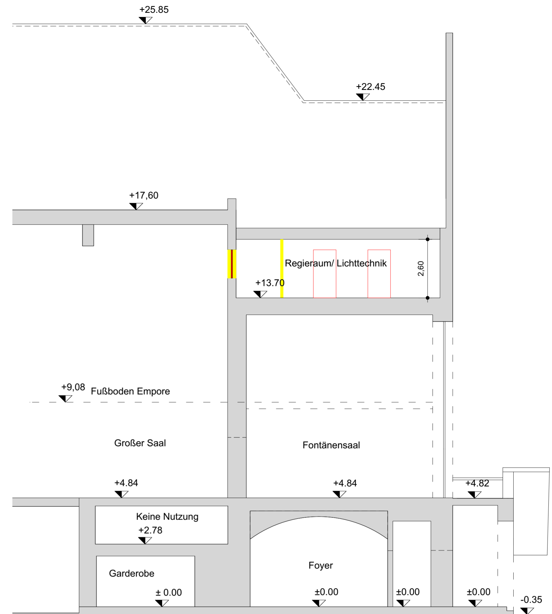
PRINZIPSCHNITT 1-1
