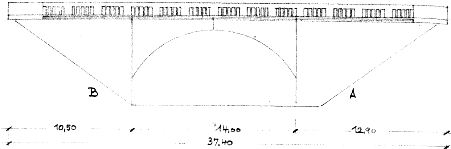
Ansicht M. 1:200
