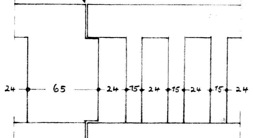
Einzelheit der Brüstung M. 1:20
