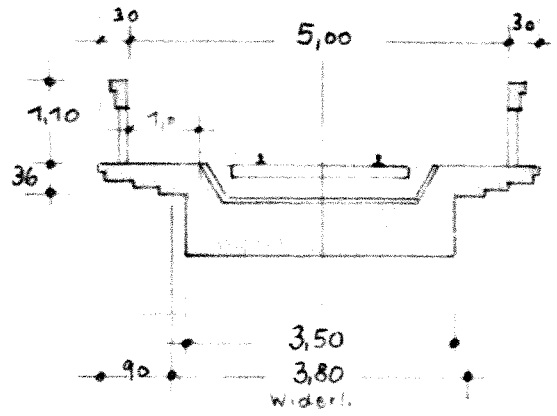
Querschnitt M. 1:100
