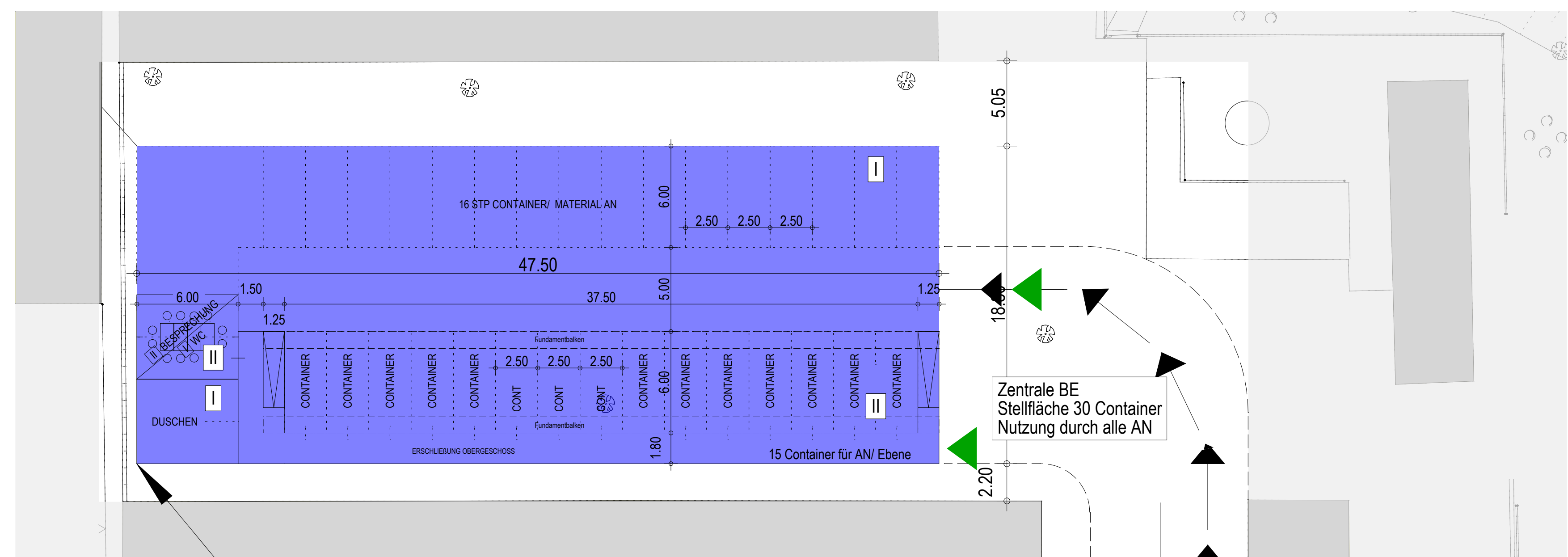
AUSSCHNITT AUFSTELLFLÄCHE CONTAINER, M 1:200
