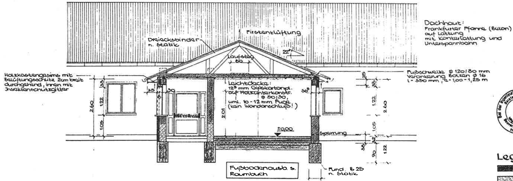
Schnitt B-B M 1:100
