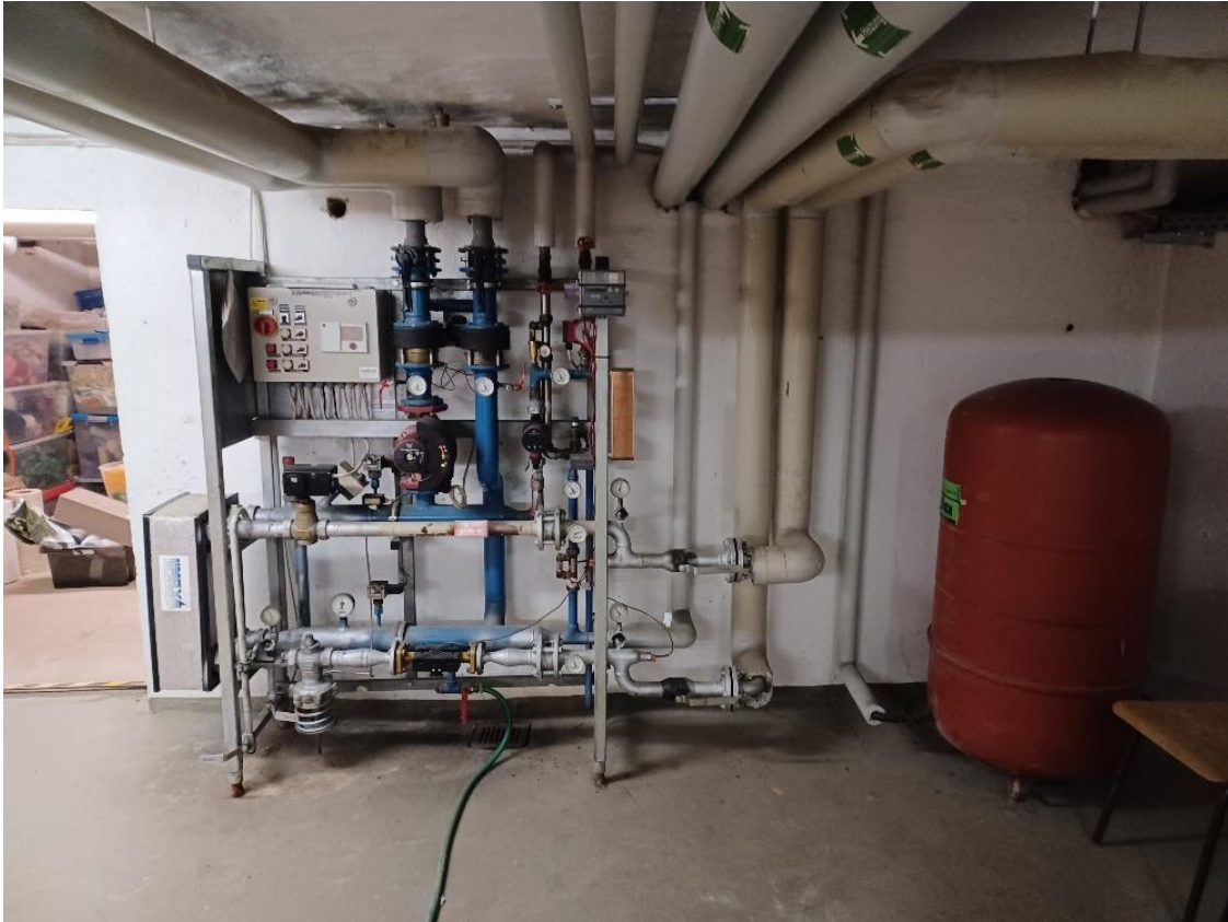
31 Hauptgebäude Keller, Fernwärmeübergabestation
