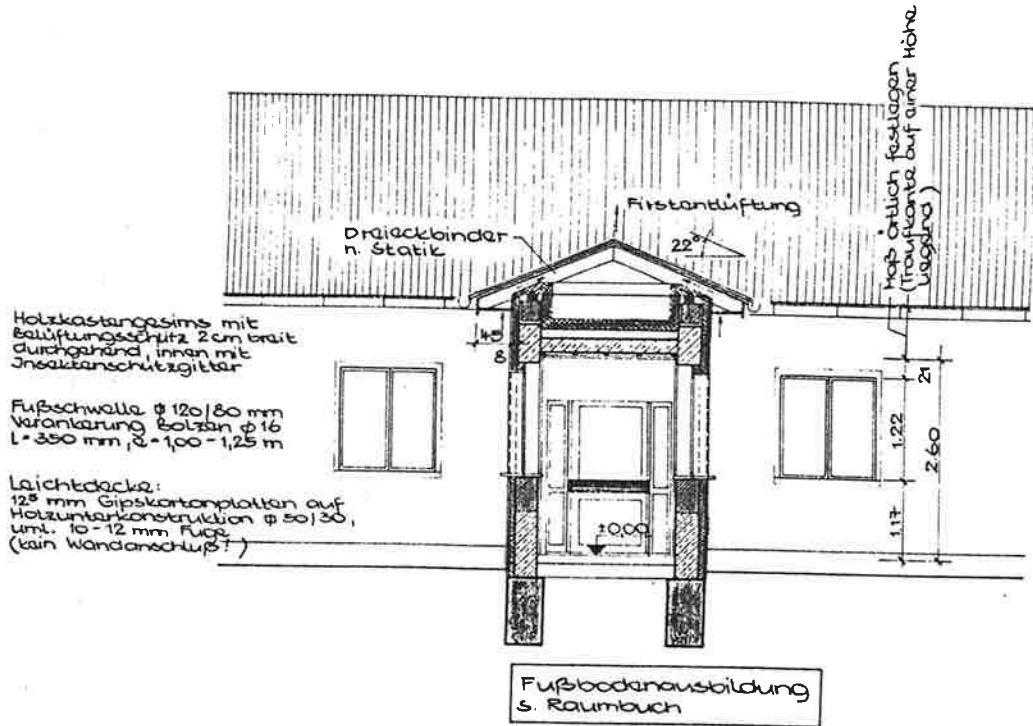
Schnitt C-C M 1:100
