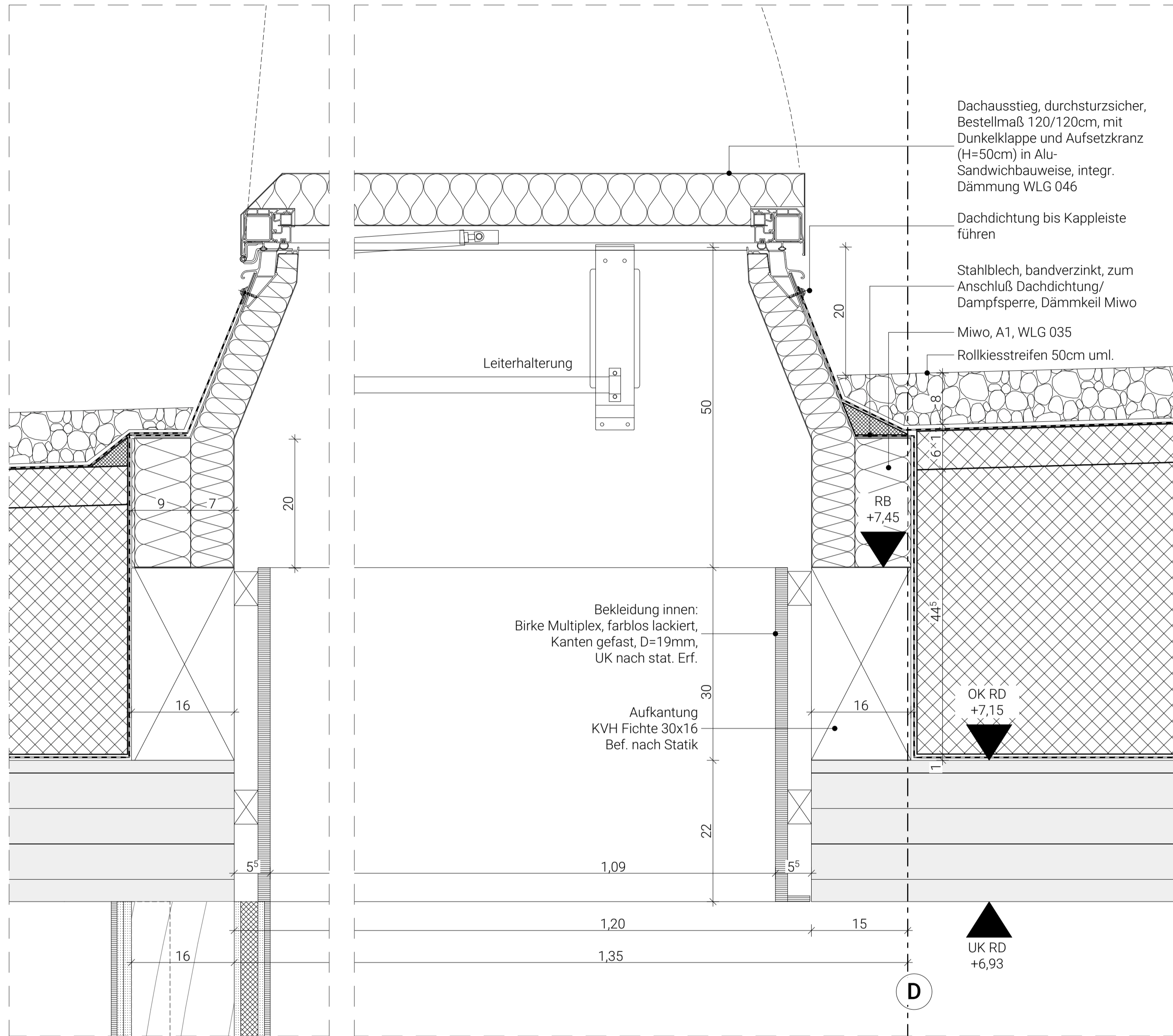
Dachausstieg M 1:5
