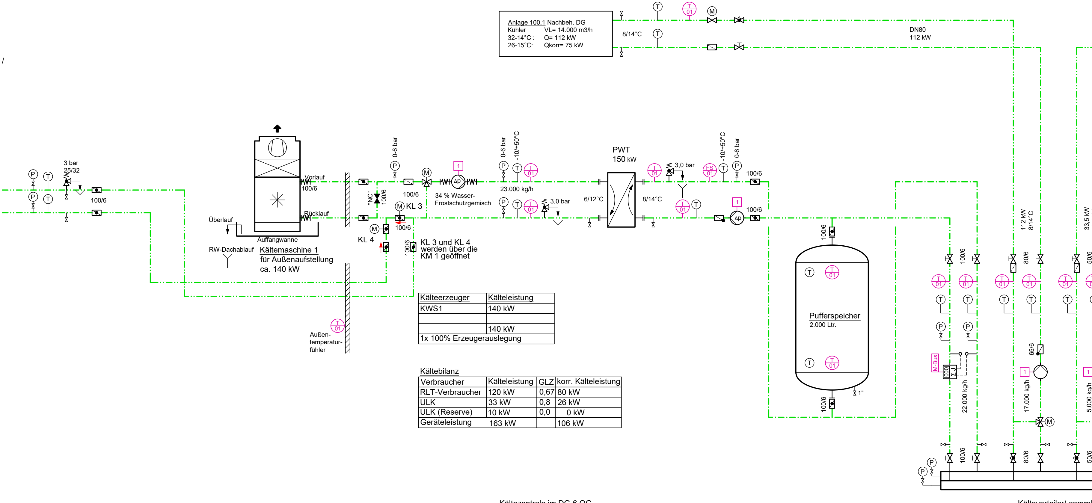
Kältezentrale im DG-6.OG
