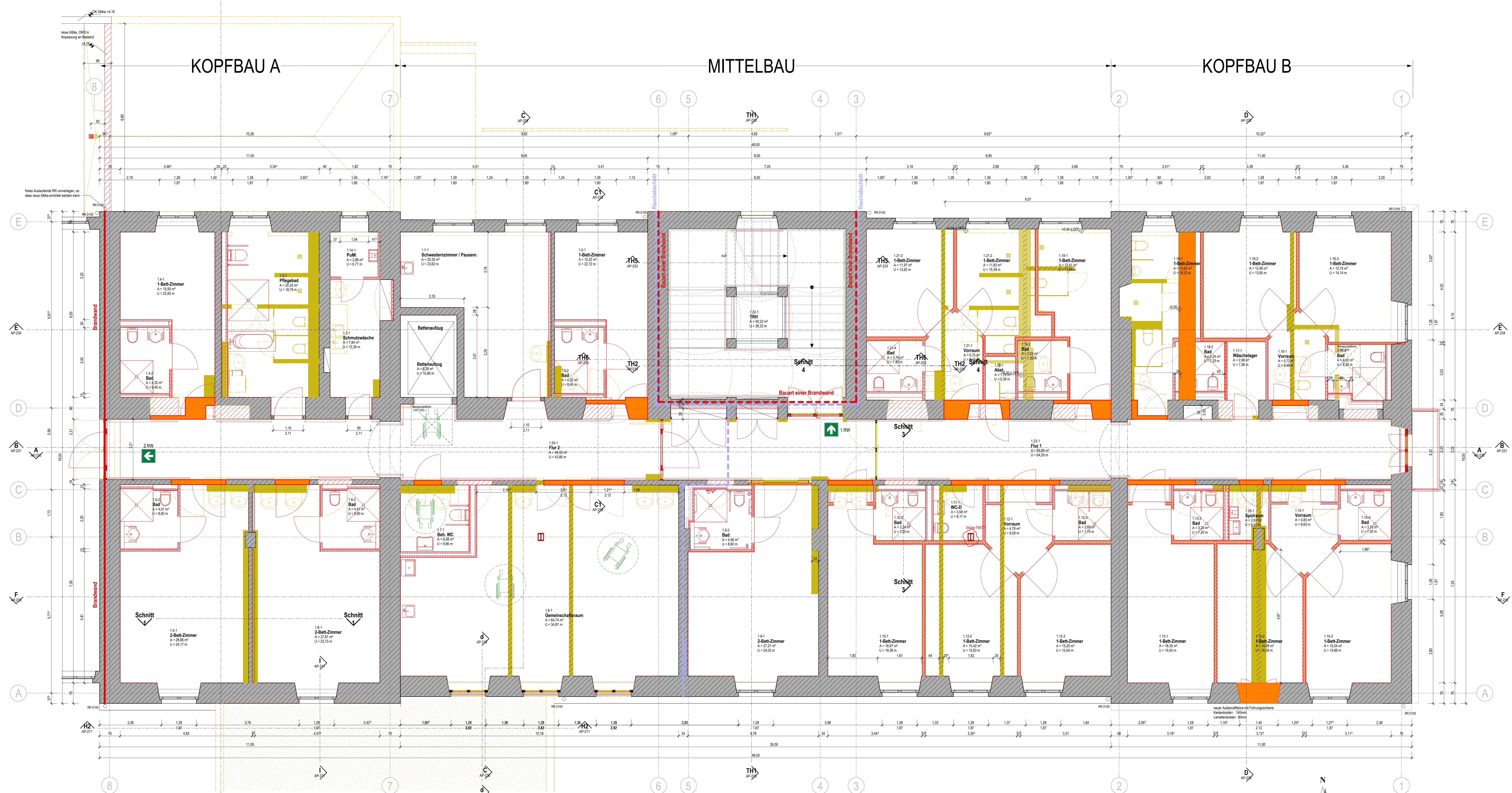
Grundriss 1.Obergeschoss Bestand, Abbruch und Neubau M 1:50
