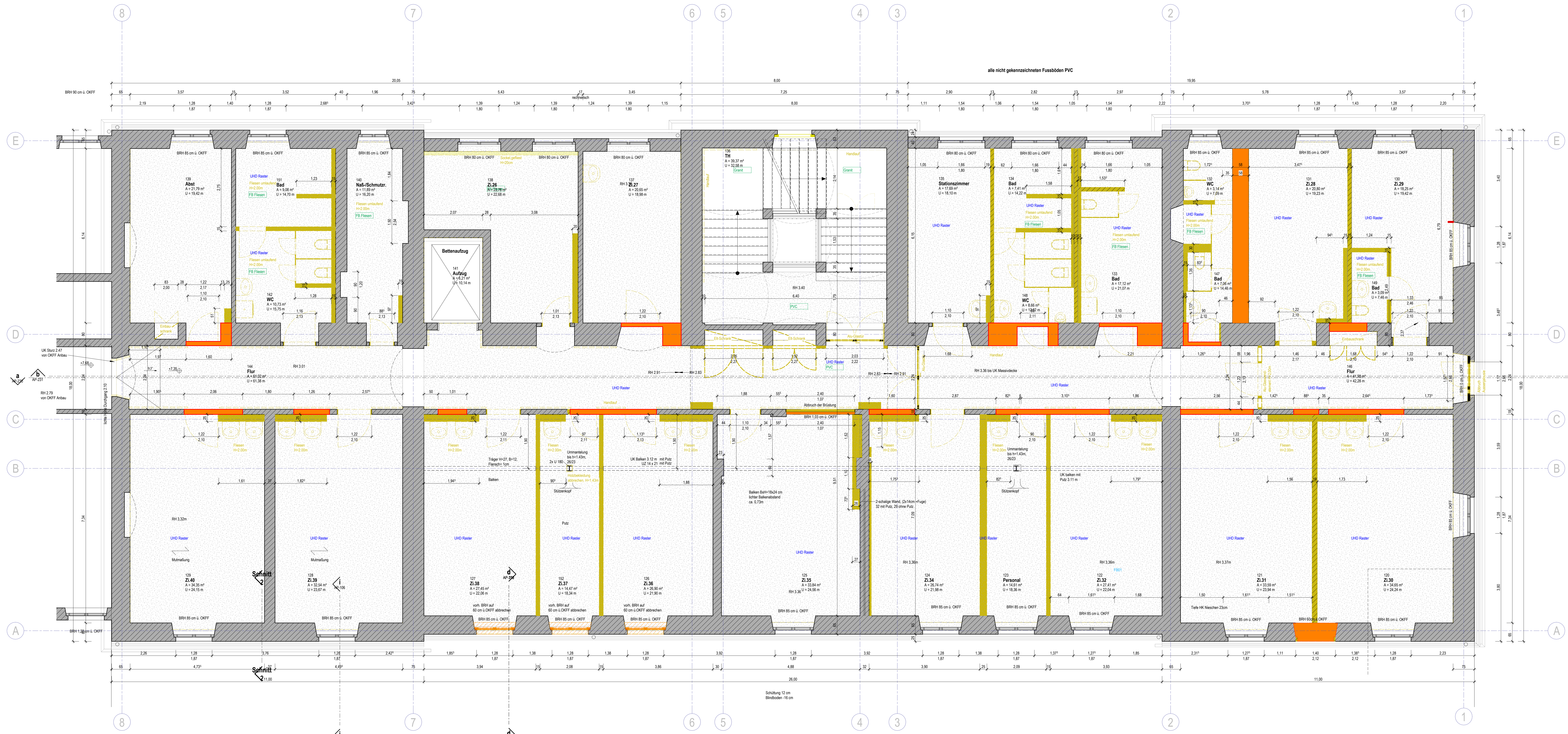
Grundriss 2.Obergeschoss Bestand und Abbruch M 1:50
