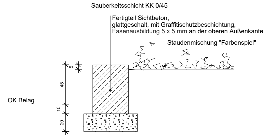
Schnitt Hochbeet schmeatisch M1:25
