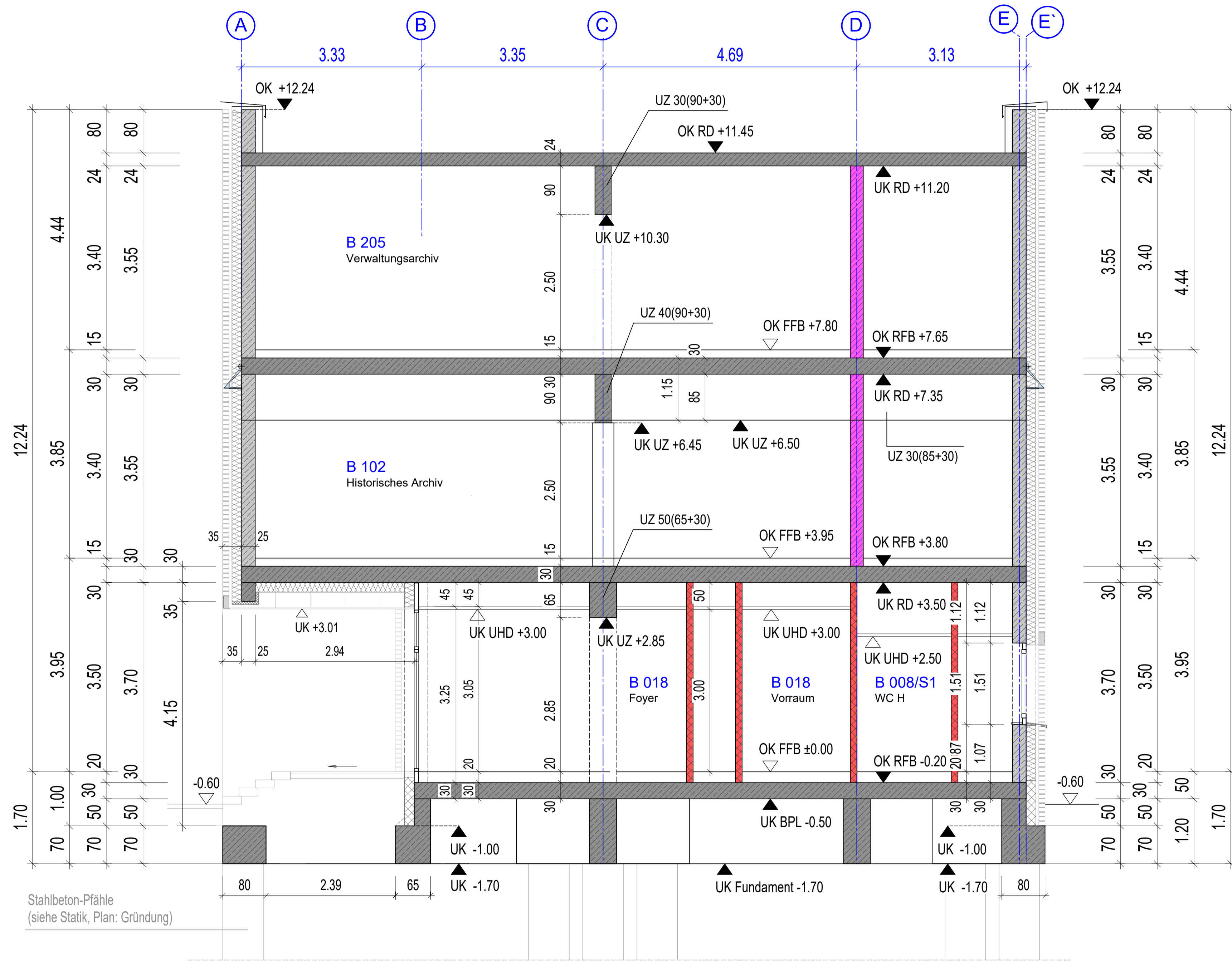
Querschnitt 7-7
