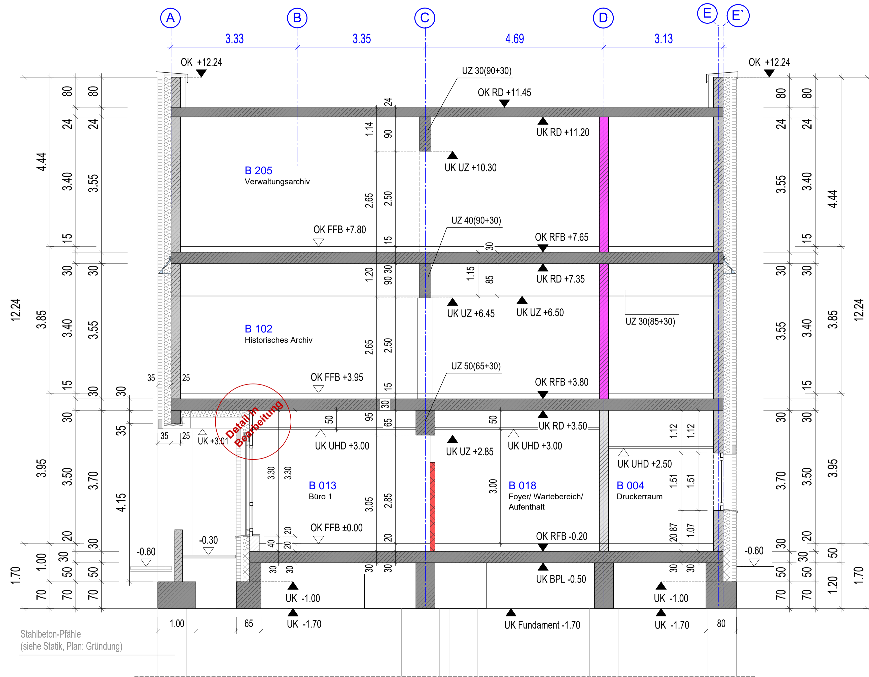
Querschnitt 6-6
