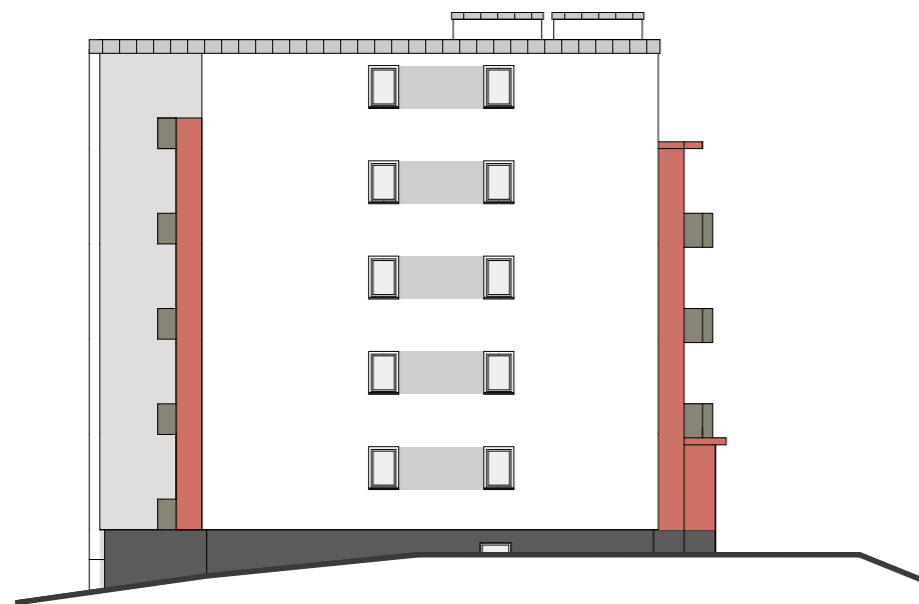
Ansicht Ostseite
