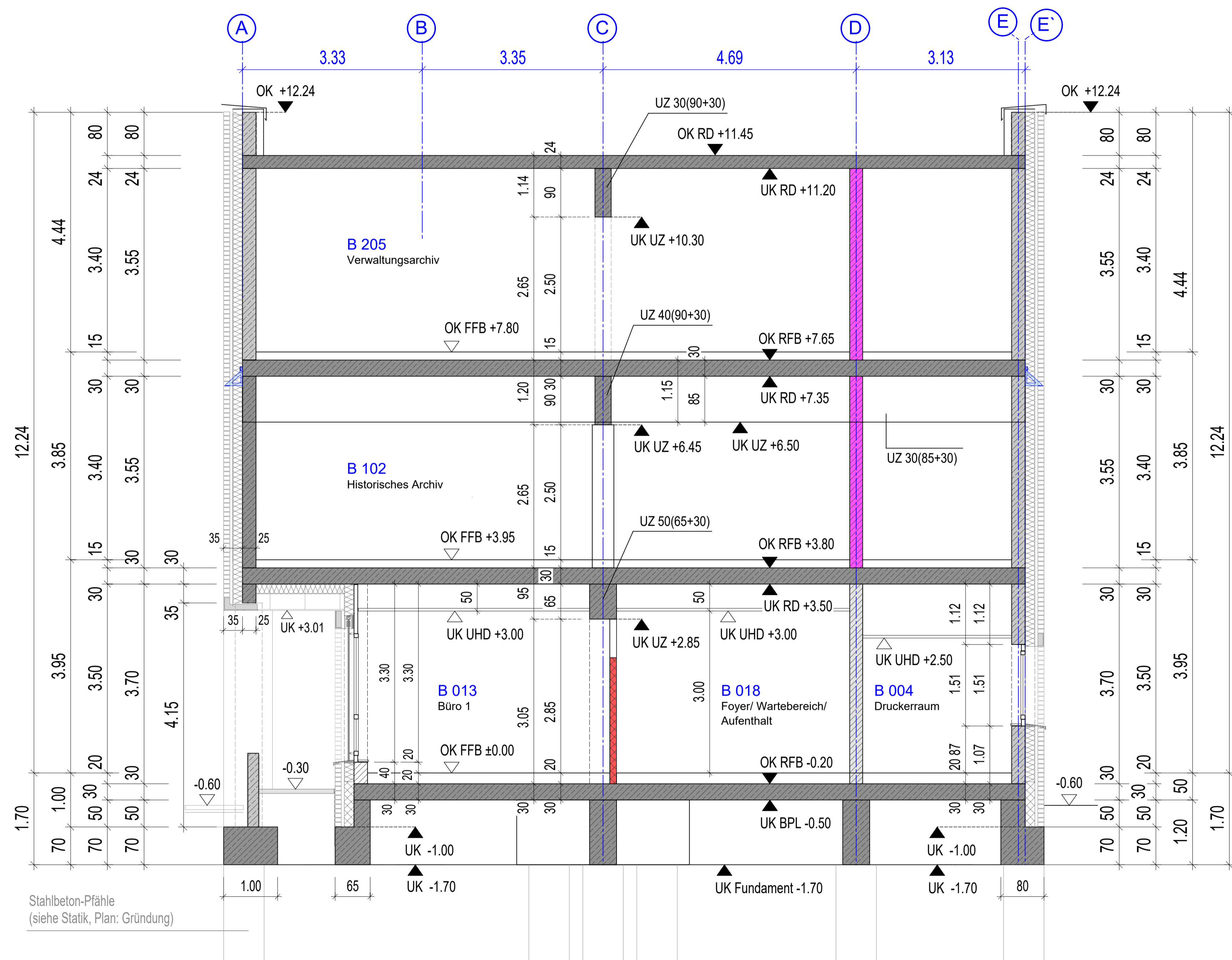
Querschnitt 6-6
