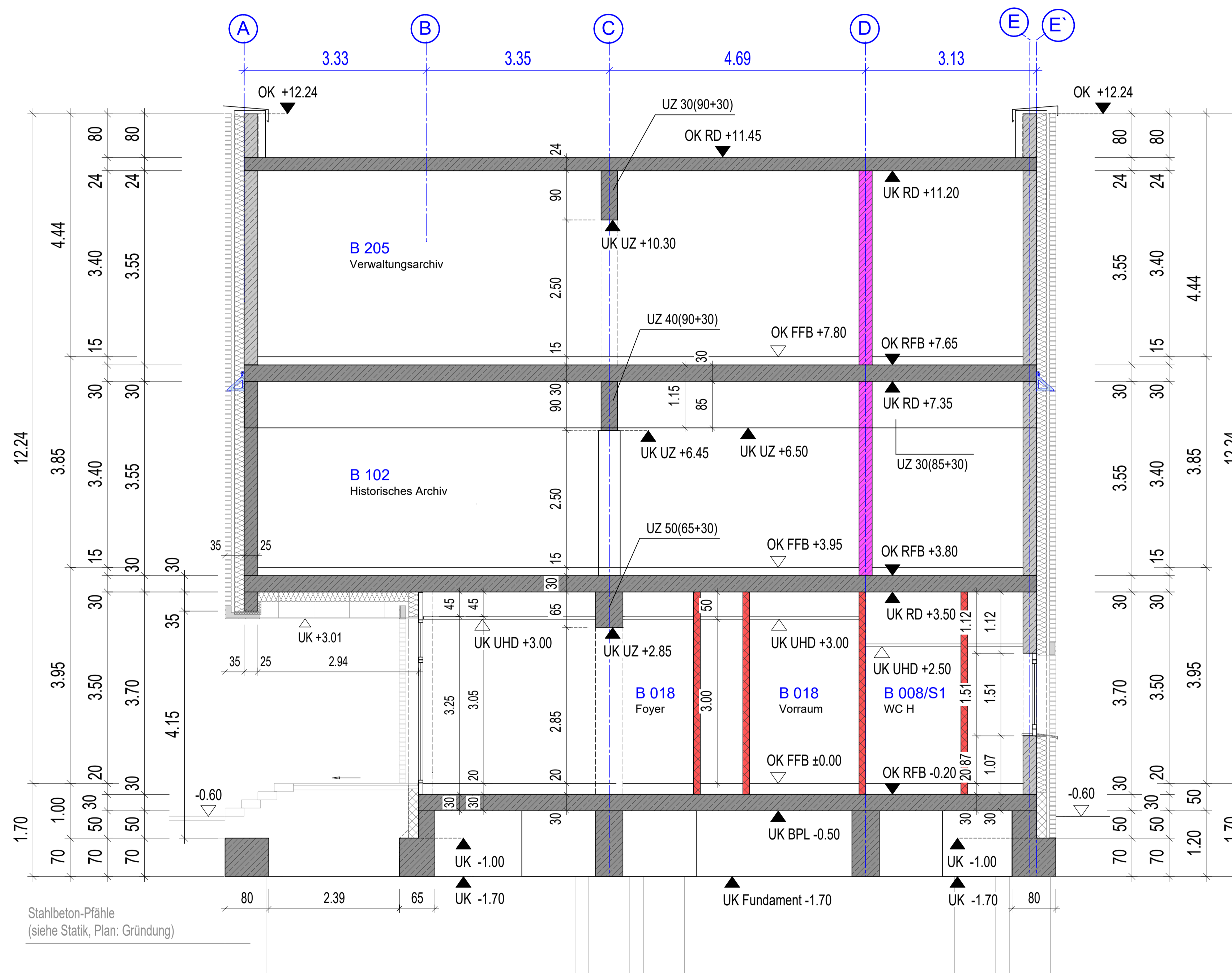
Querschnitt 7-7
