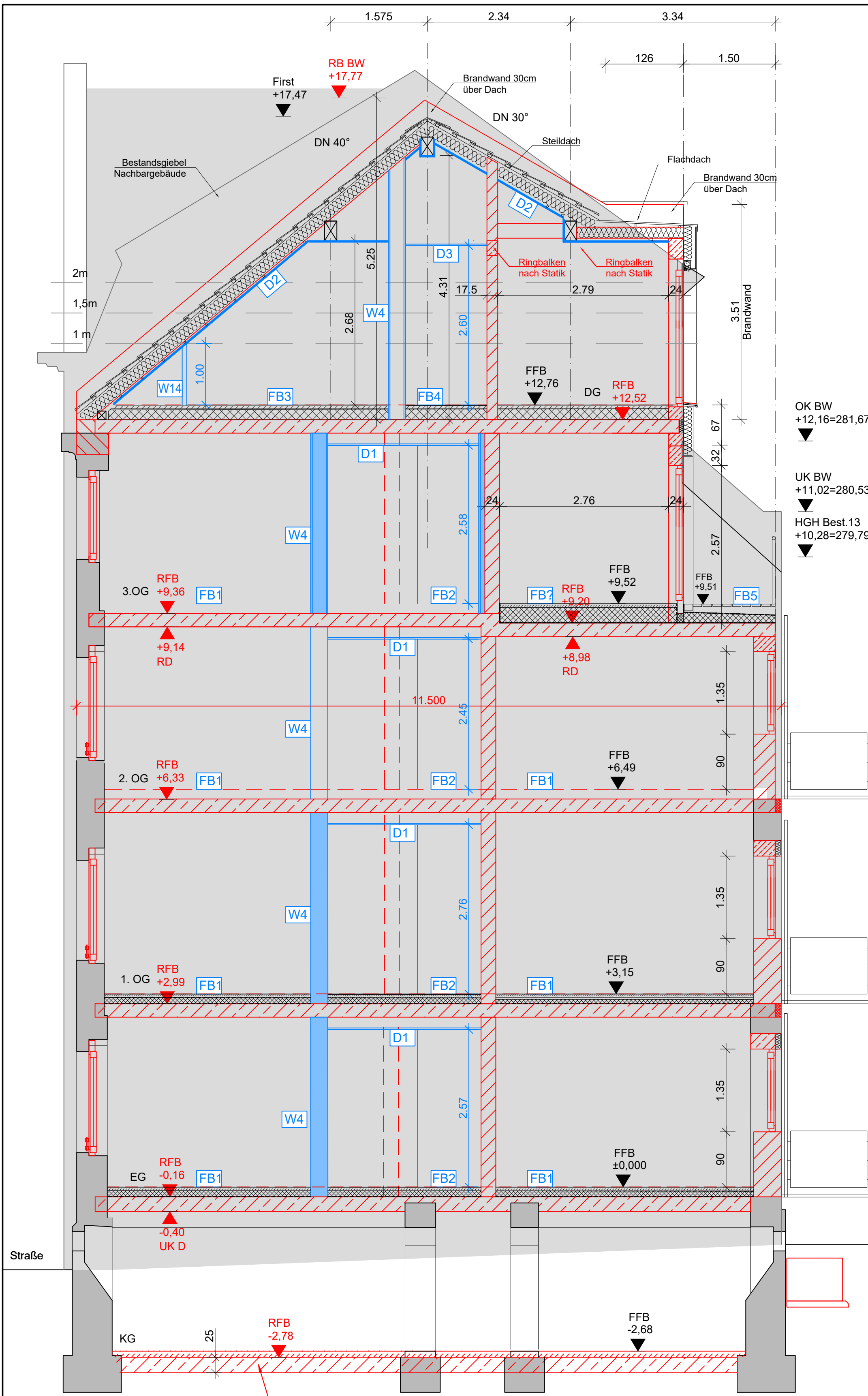
Schnitt E-E Nr.13
