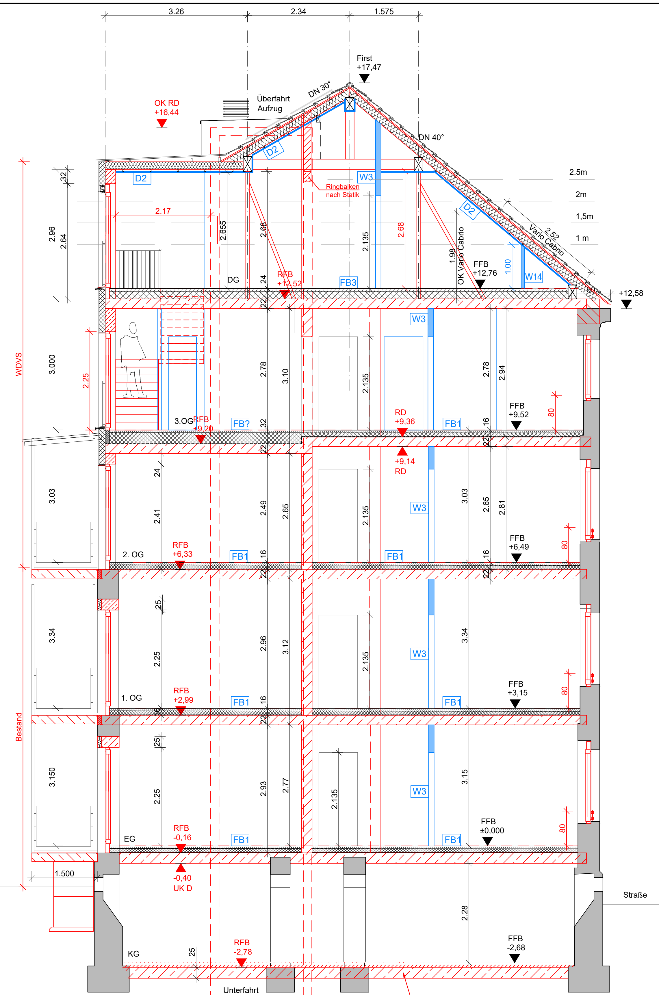
Schnitt B-B Nr.13
