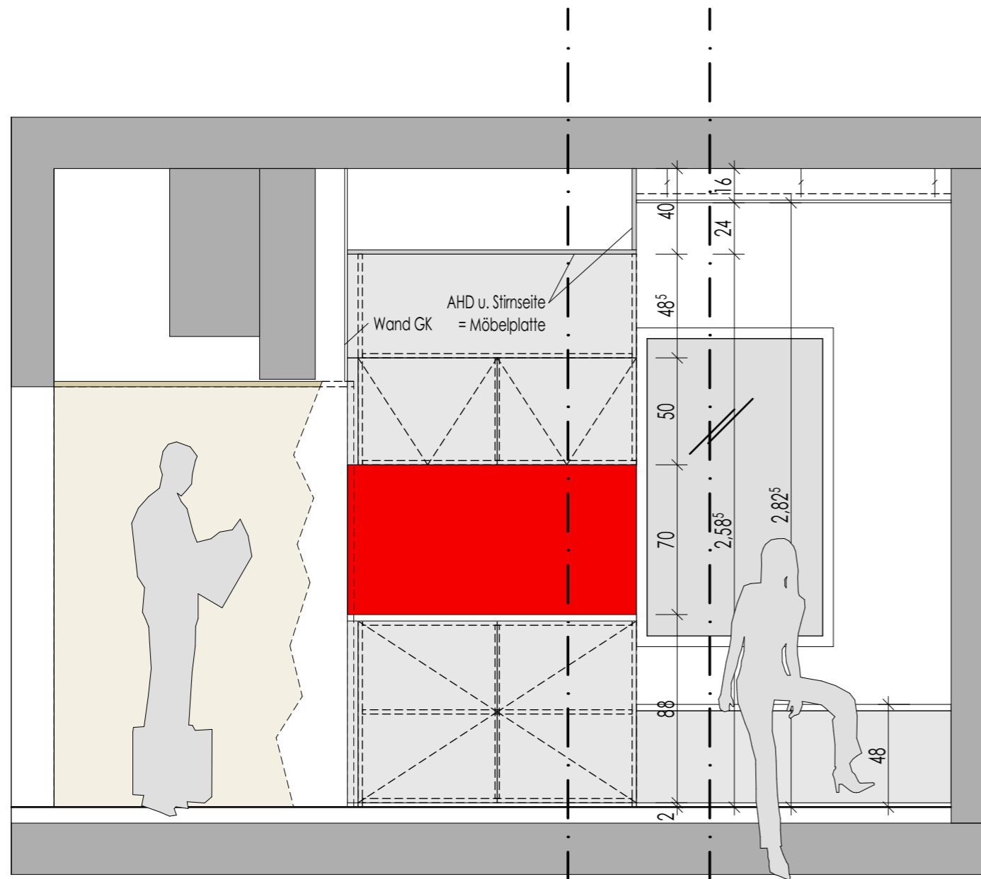
Ansicht rechts b-b
