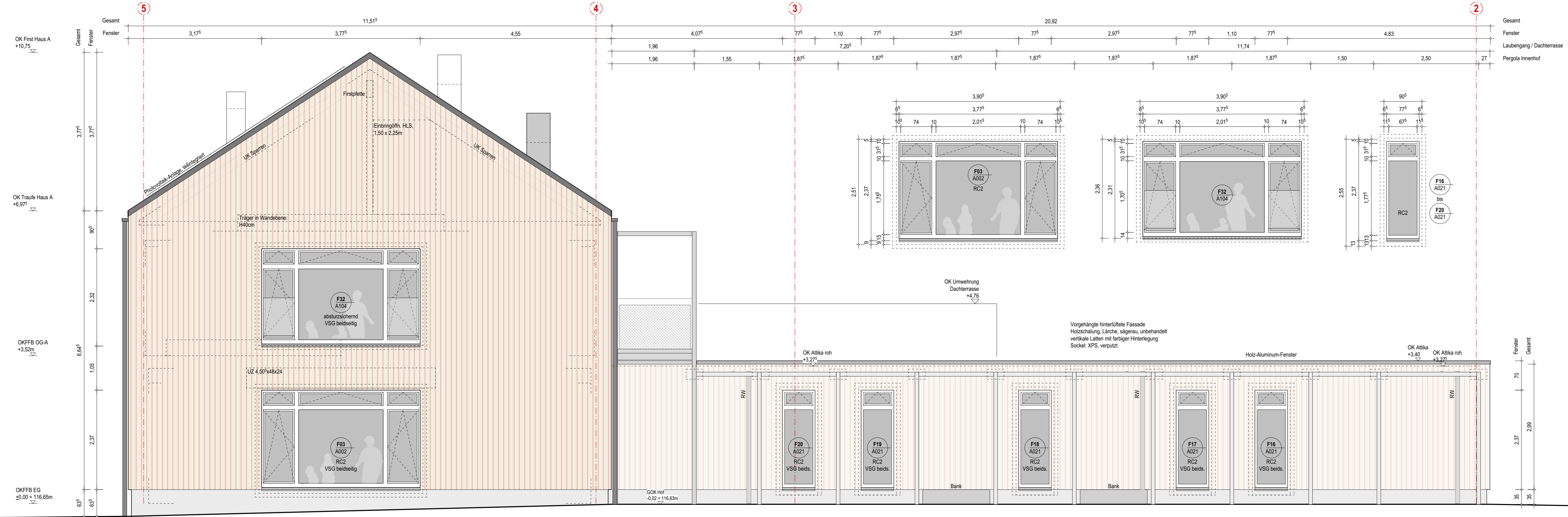
A-N: HAUS A, Ansicht von Norden
