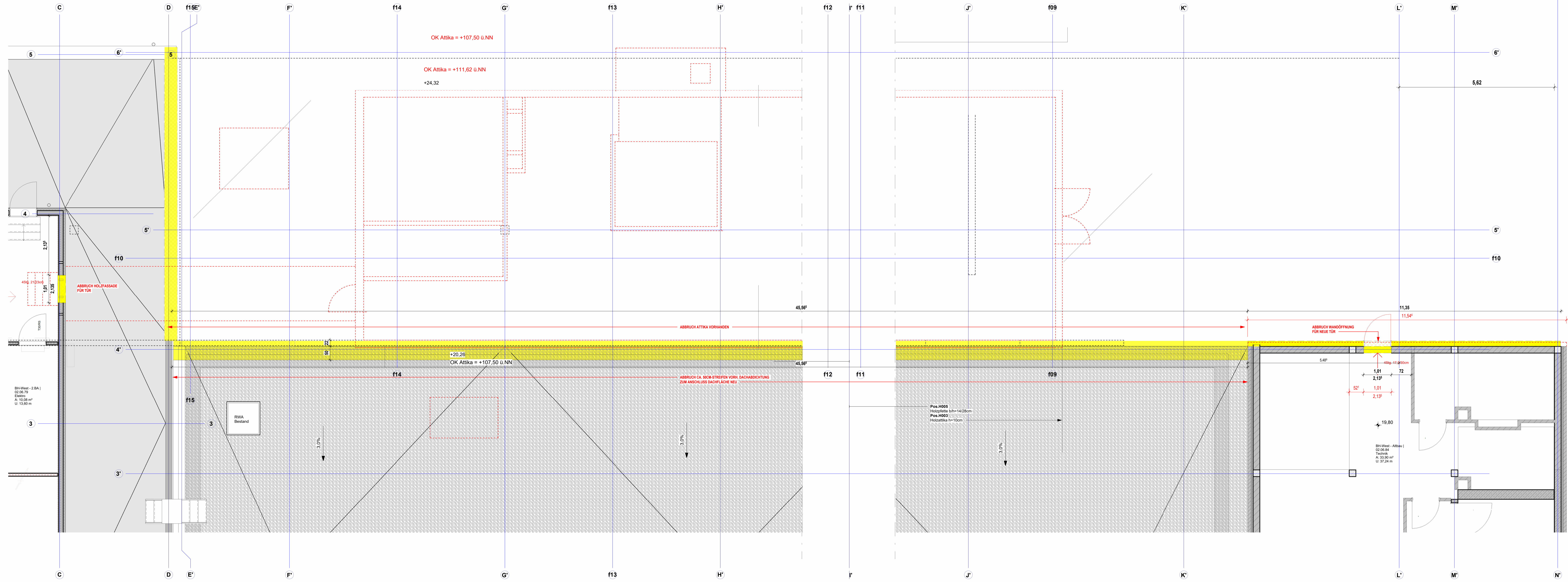
6. Obergeschoss - Rohbau - Abbruchplan M. 1:50
