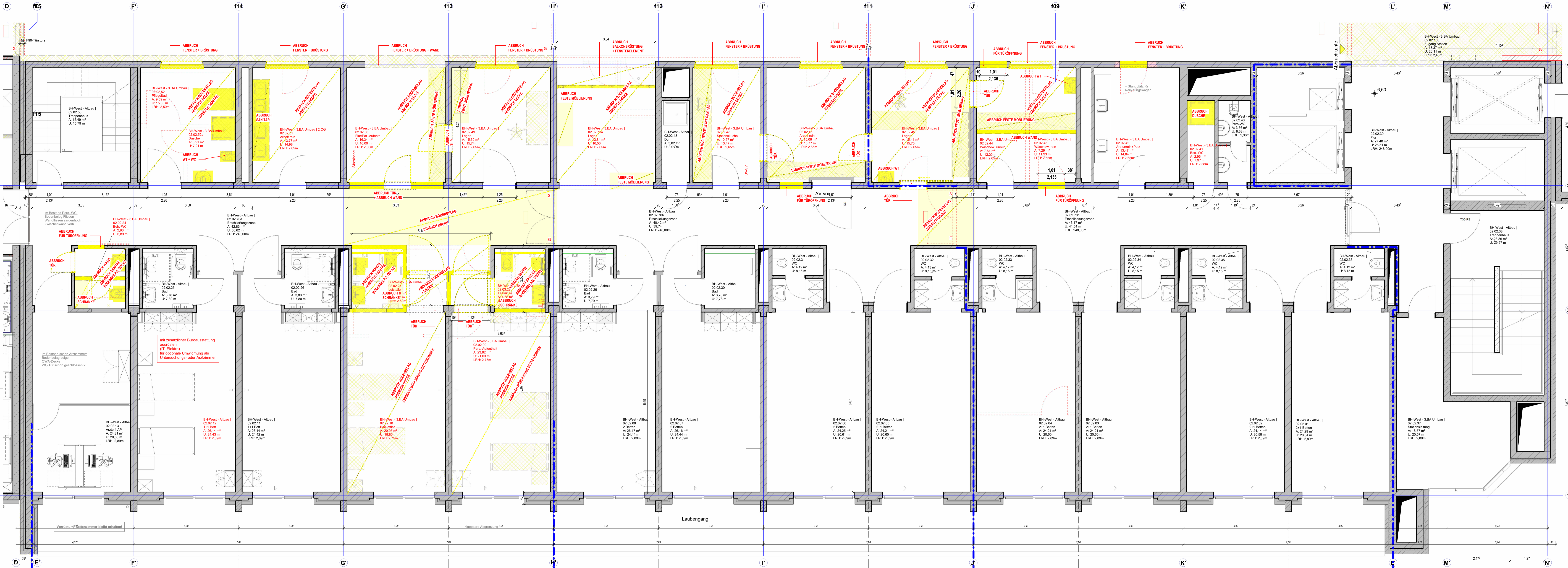
2. Obergeschoss - Rohbau - Abbruchplan M. 1:50
