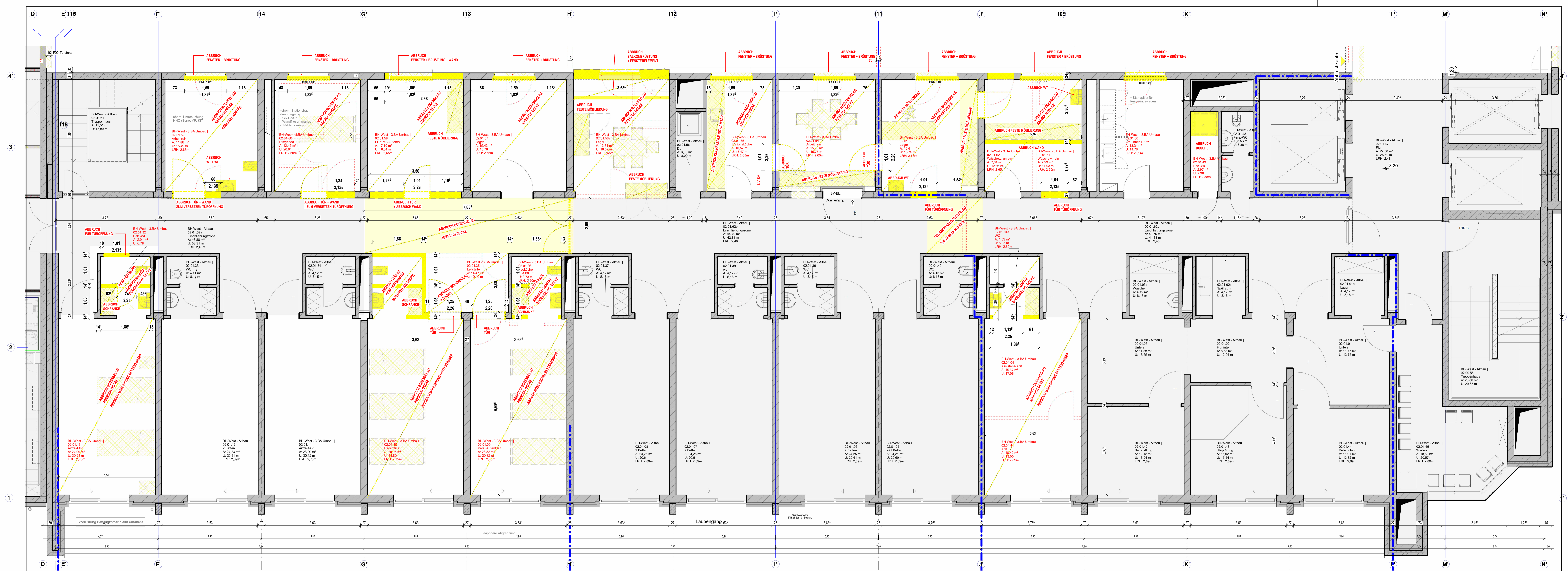
1. Obergeschoss - Rohbau - Abbruchplan M. 1:50
