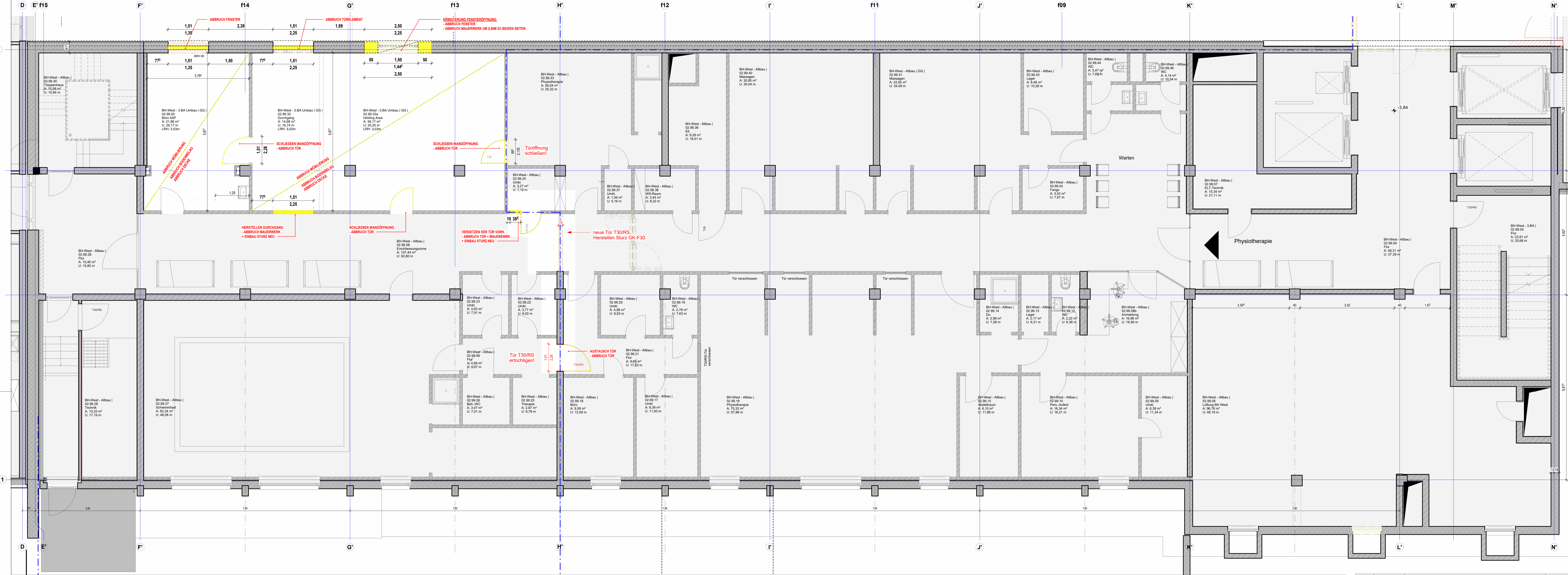
Gartengeschoss - Rohbau - Abbruchplan M. 1:50
