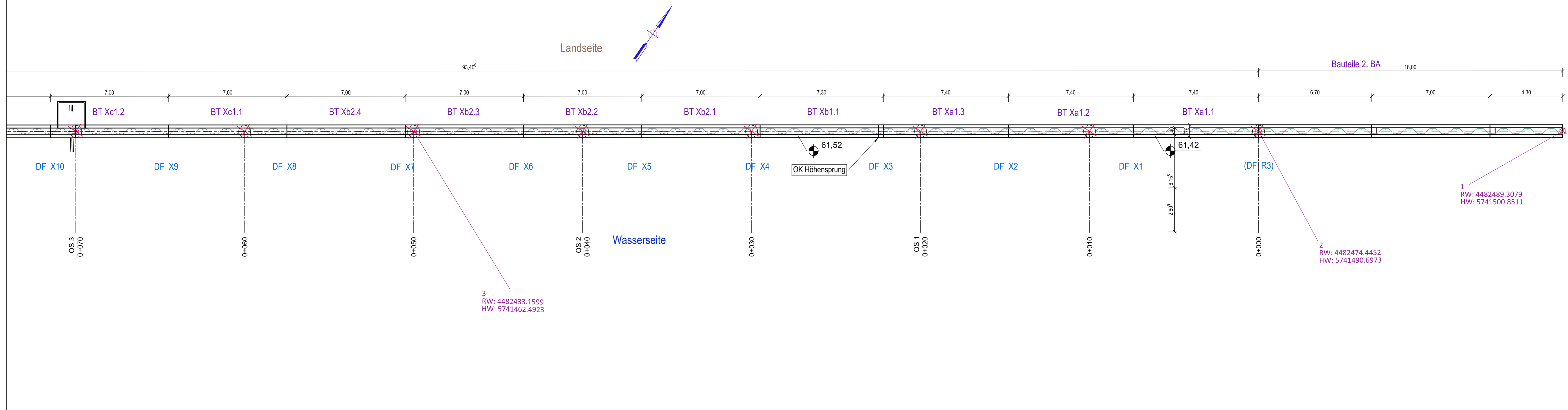
Grundriss Abschnitte, Bauteile (Anfang) BT Xa1.1 bis BT Xc1.2 (Station 0+ 0,0 bis Station 0+70,0) M 1:100
