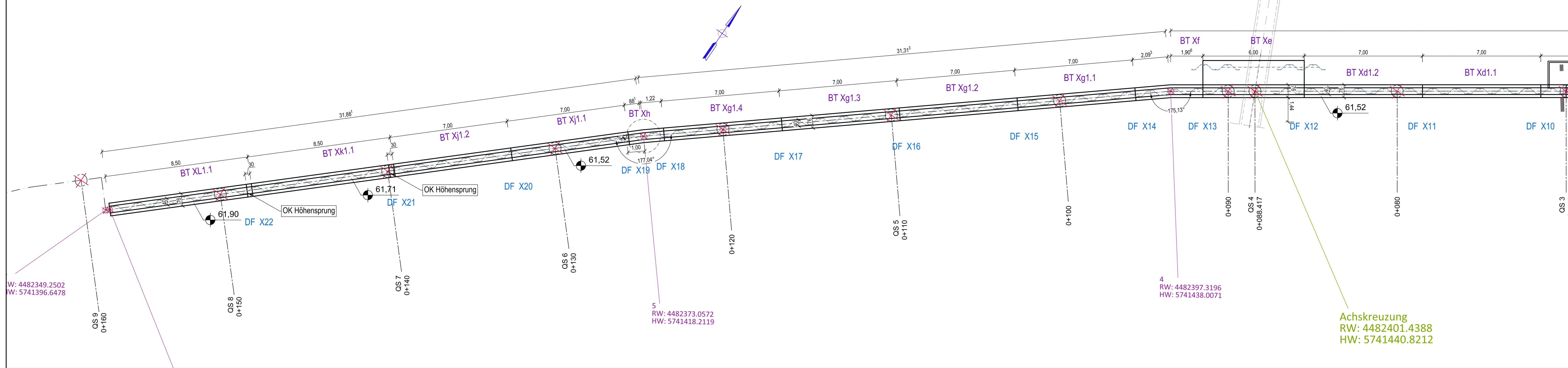
Grundriss Abschnitte, Bauteile BT Xd1.1 bis BT XI1.1 (Ende Station 0+ 70,0 bis Station 0+160,0) M 1:100
