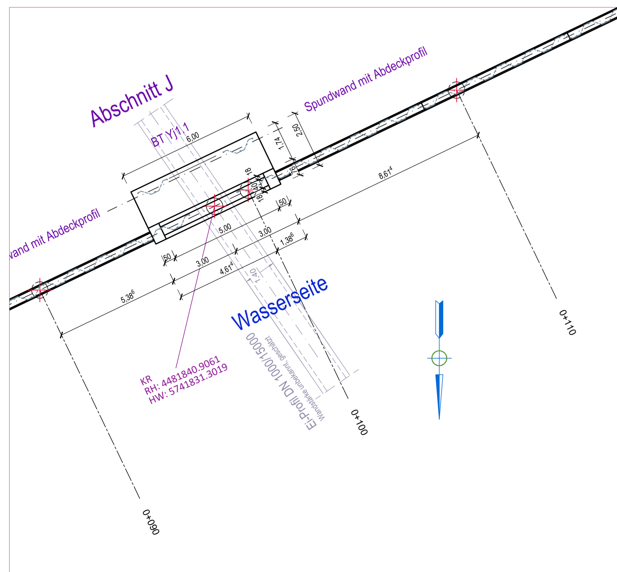
Grundriss Abschnitt J, Bauteil BT Yj 1.1 (Kanalquerung) M 1:100
