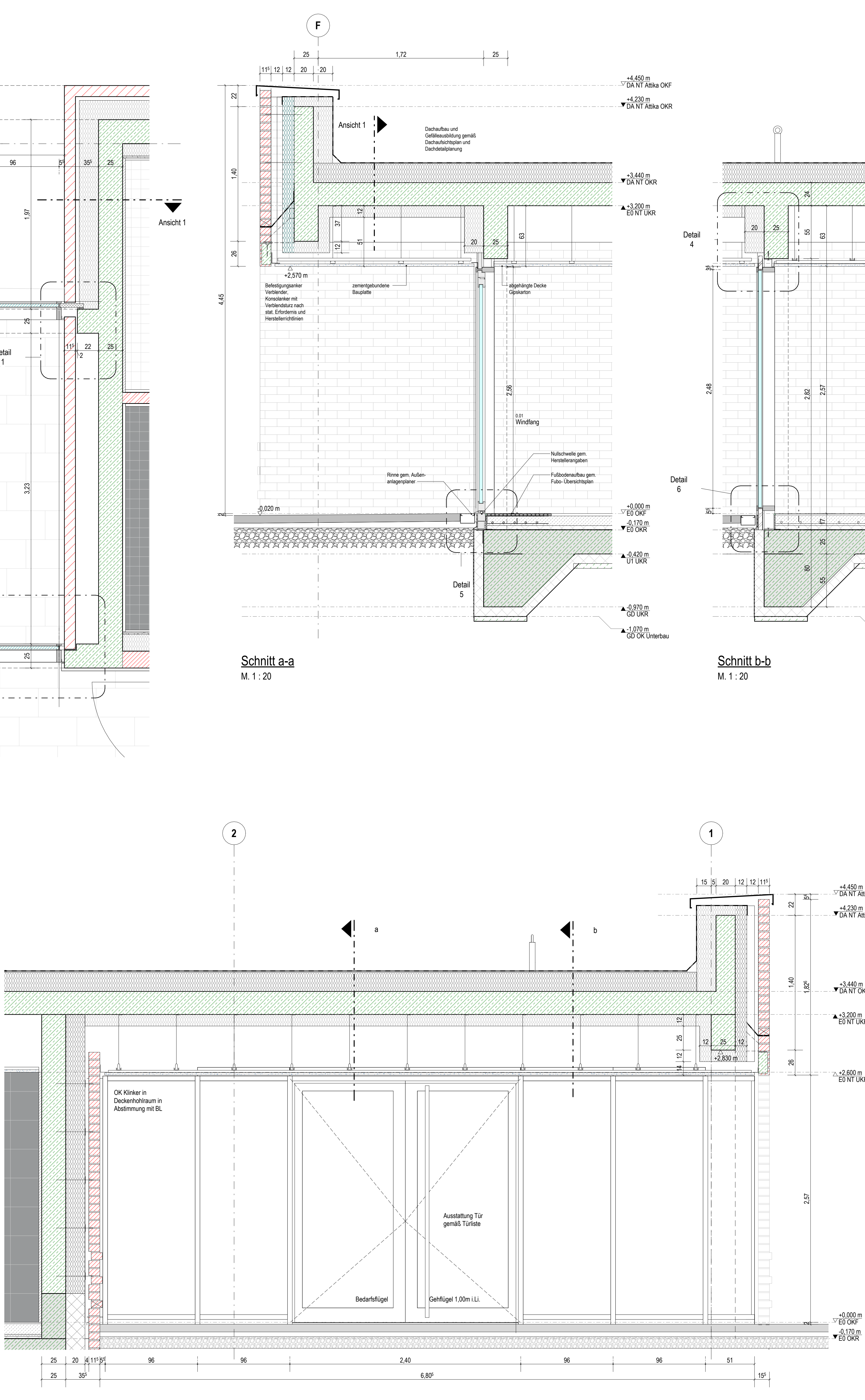
Schnitt a-a M. 1: 20
