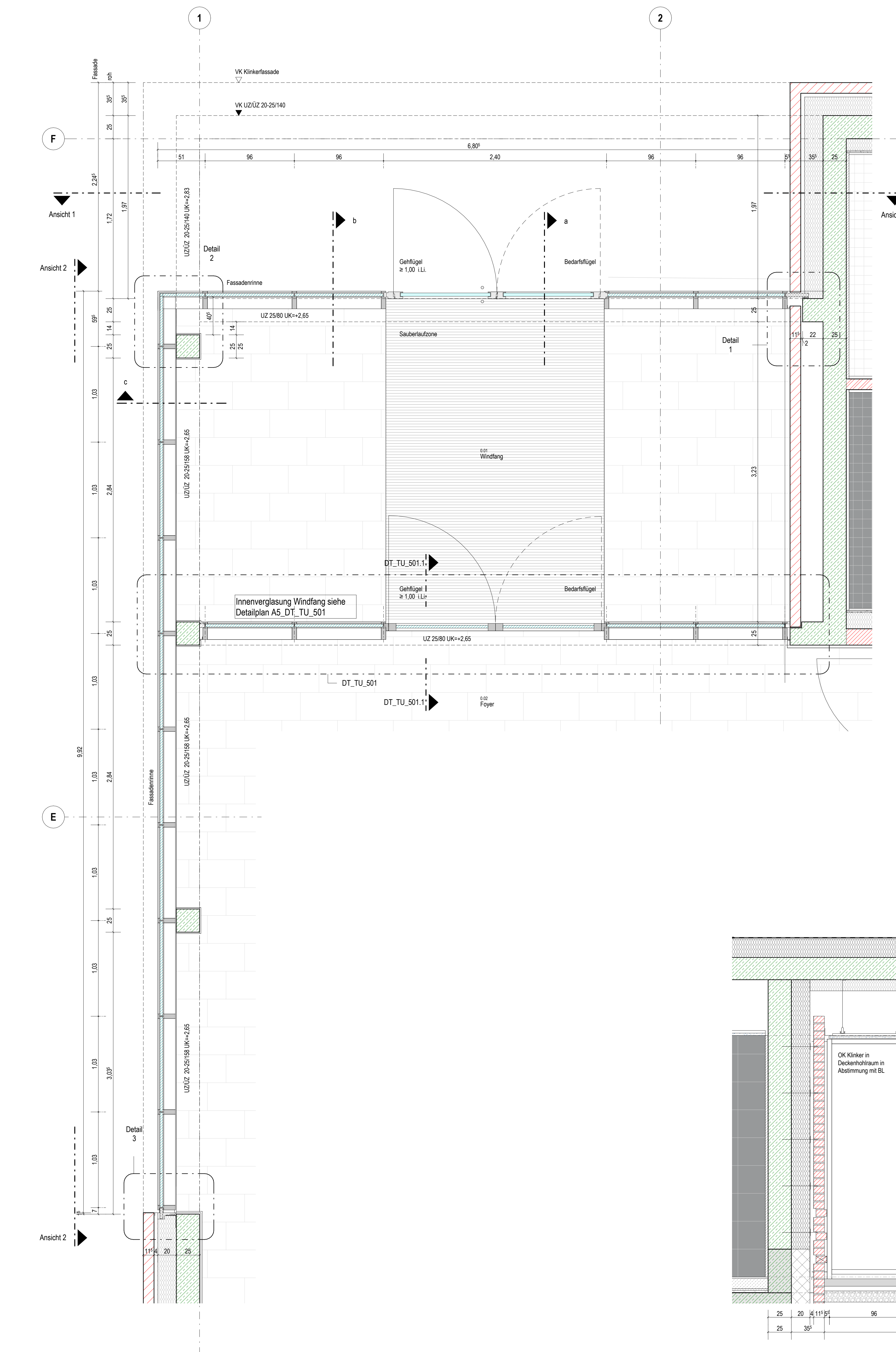
Grundriss M. 1: 20
