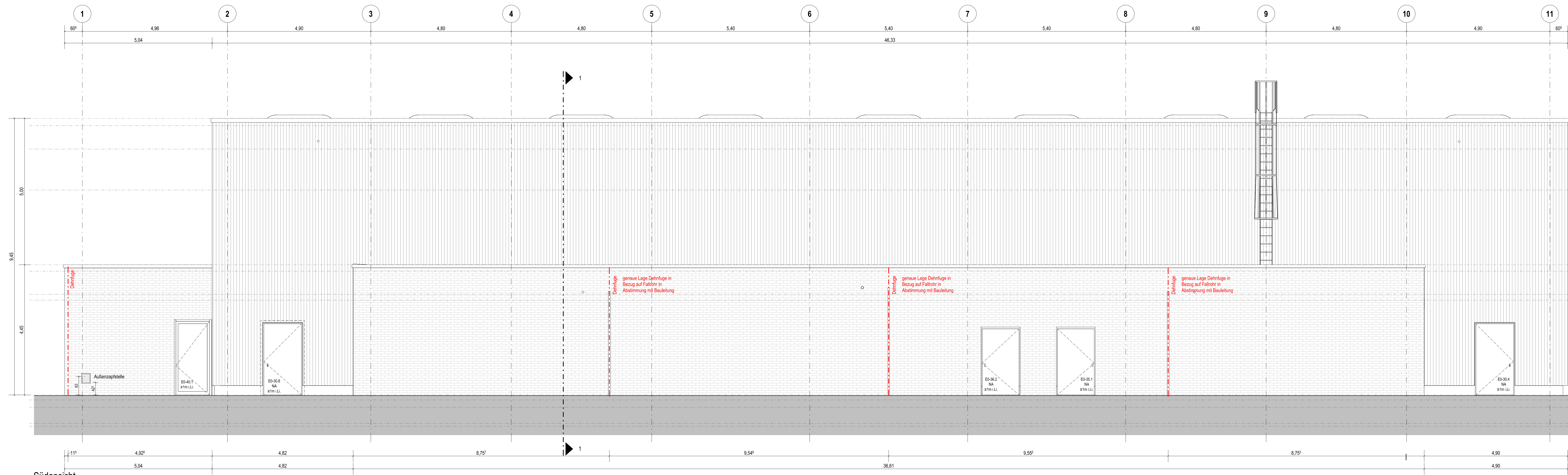
Südsansicht
