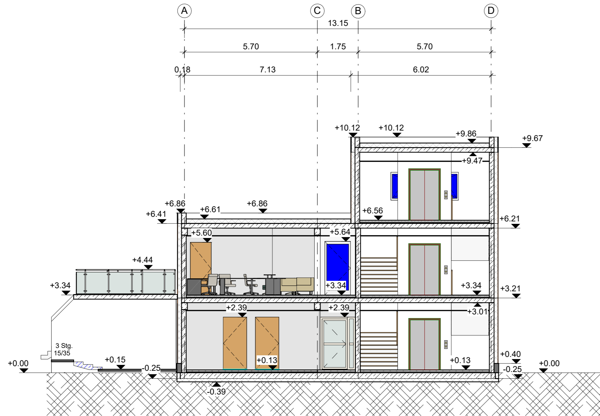
Schnitt 1-1 Multifunktionsgebäude 1:100
