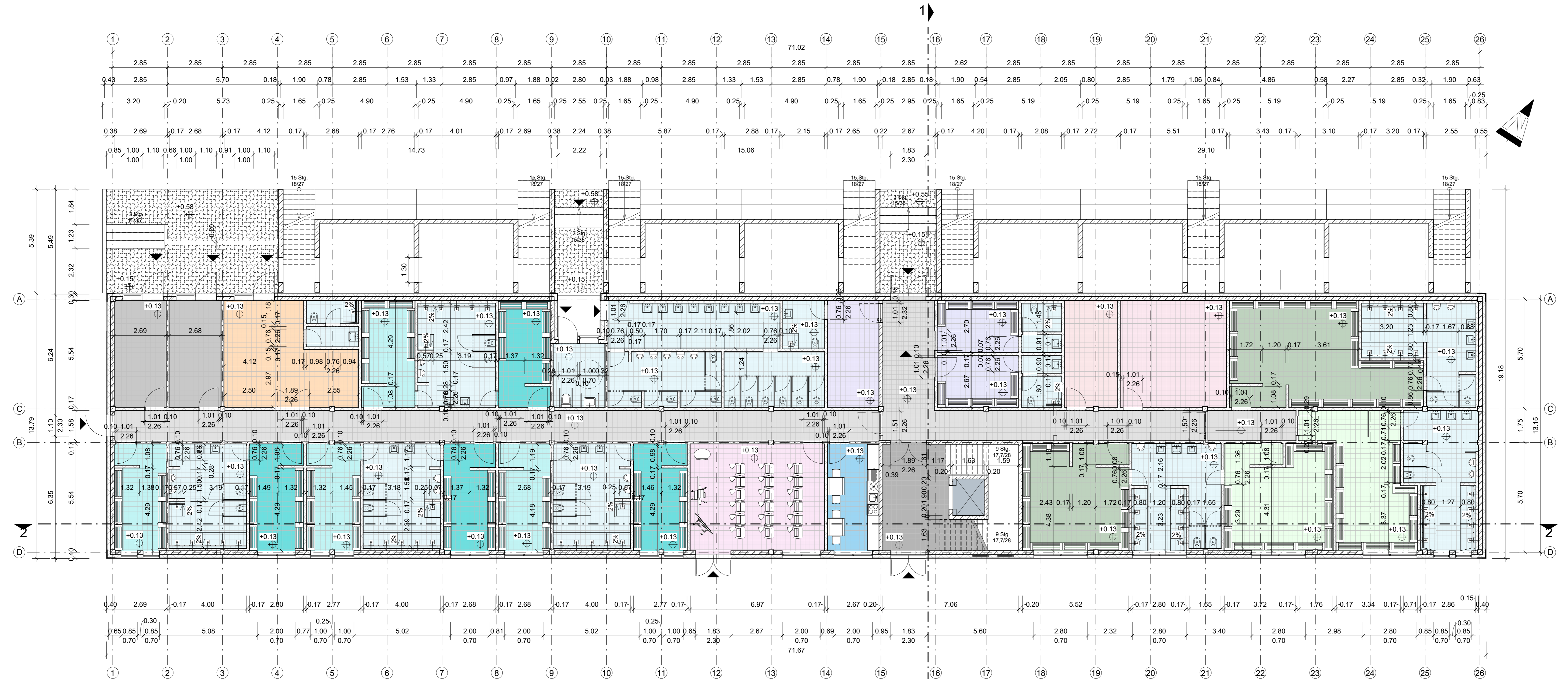
Grundriss Erdgeschoss Multifunktionsgebäude 1:100
