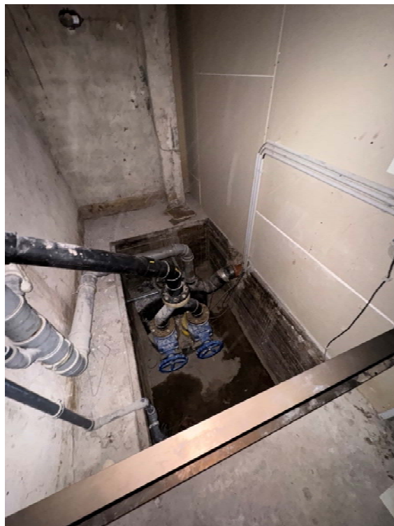
Nr. 9 Hebeanlage
