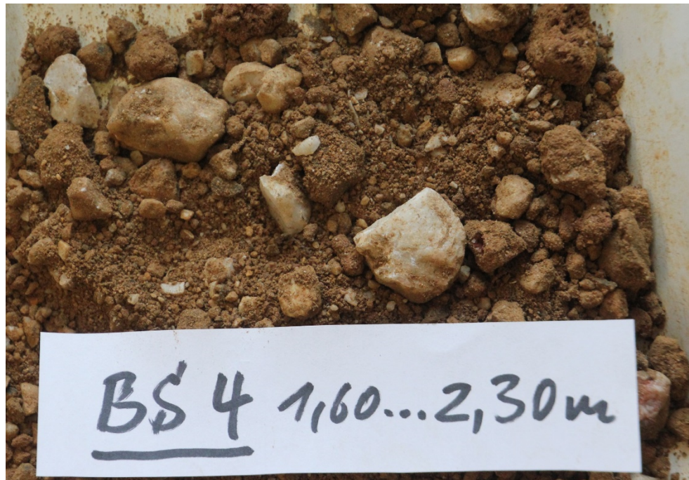
Foto 28: Bohrung BS 4 – Bohrkern 1,60...2,30 m/ Tertiäre Kiessande
