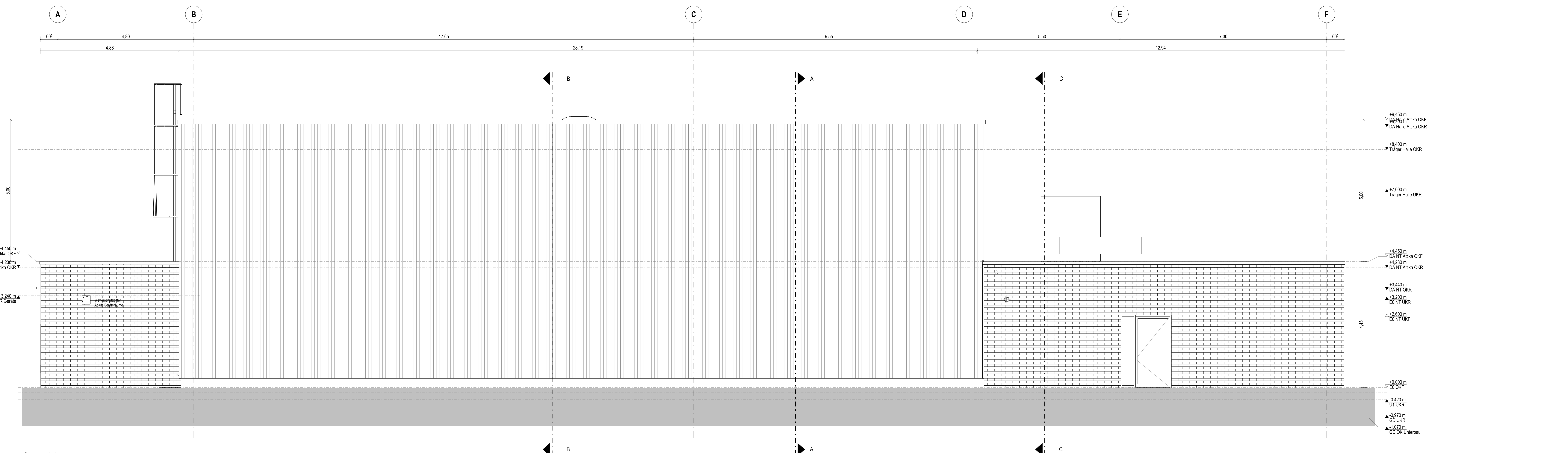
Ostansicht
