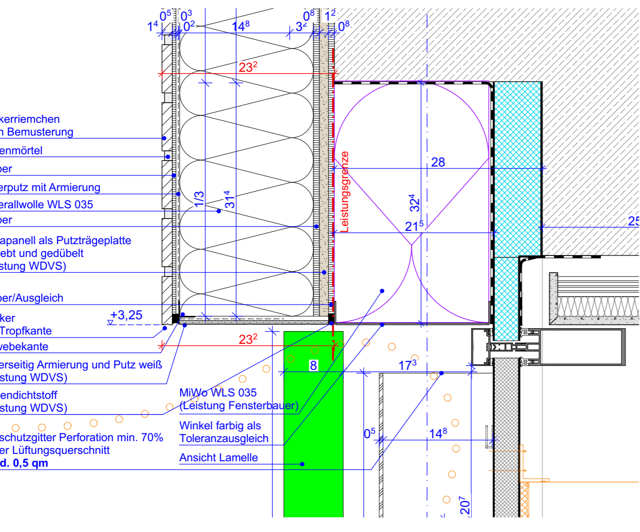
SCHNITT 1
