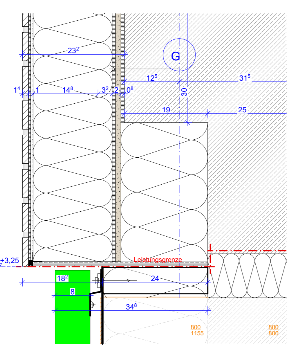
SCHNITT 6
