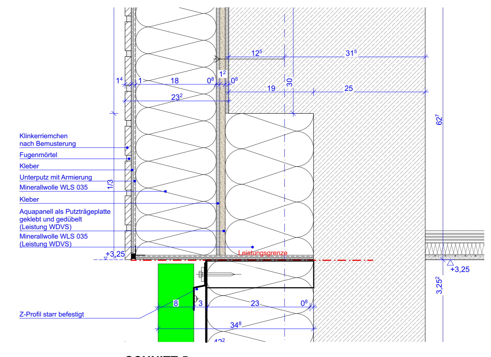
SCHNITT 5
