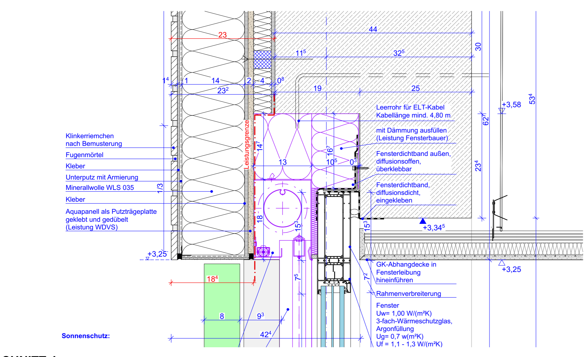
SCHNITT 4
