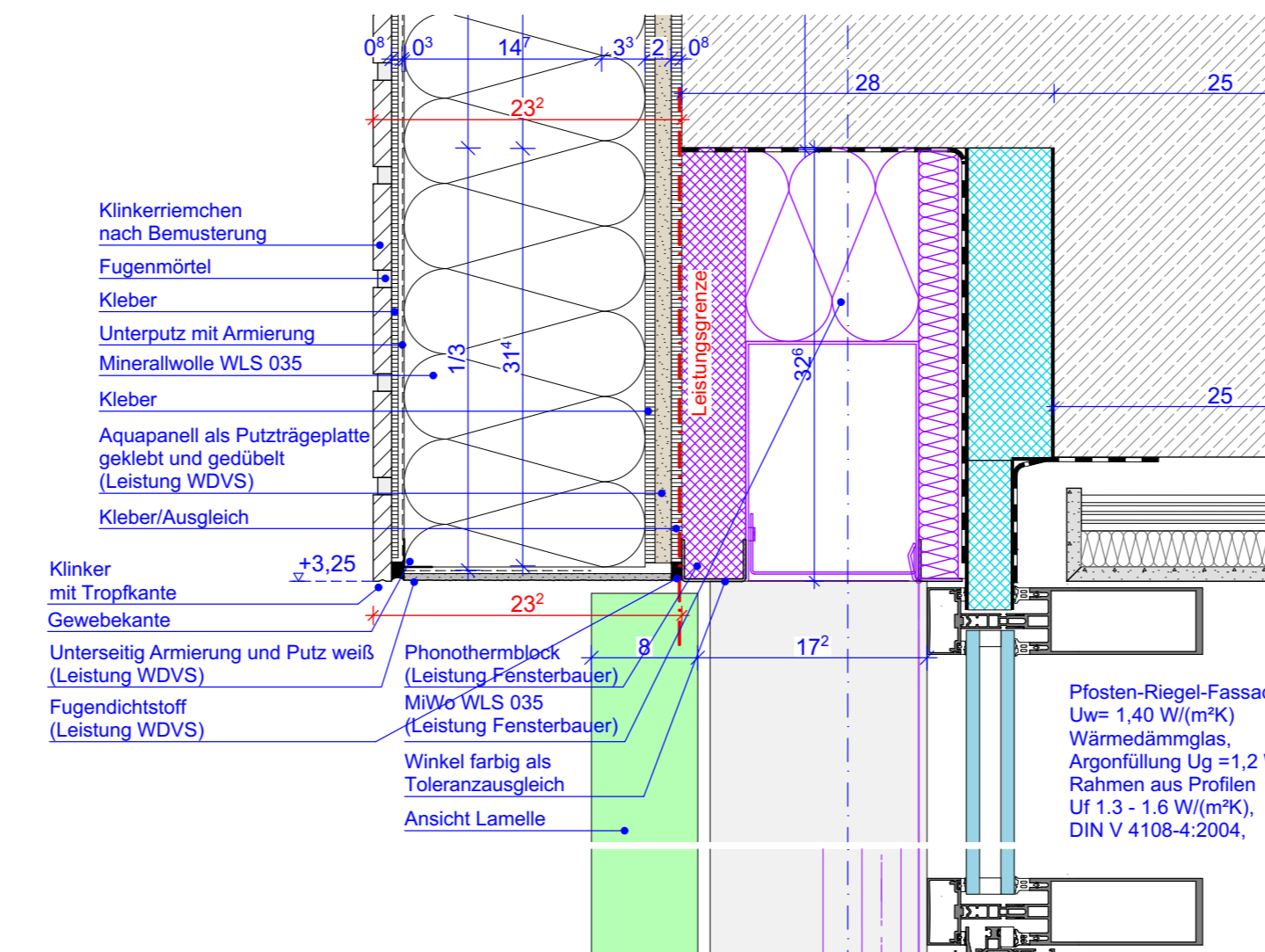
SCHNITT 2.2
