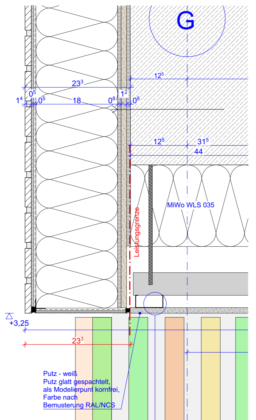
SCHNITT 7
