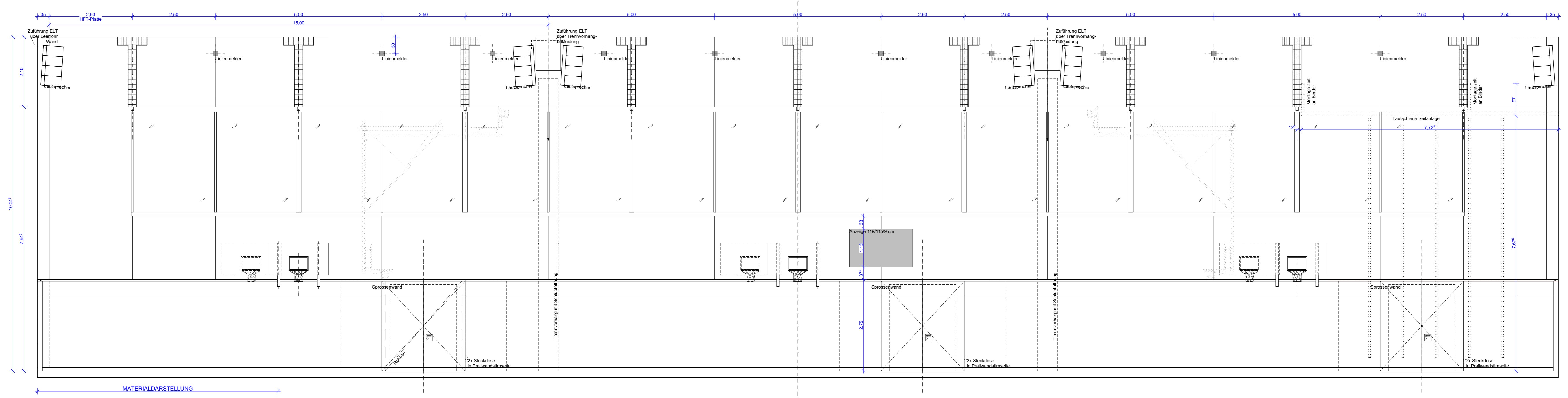
Wandabwicklung Achse A
