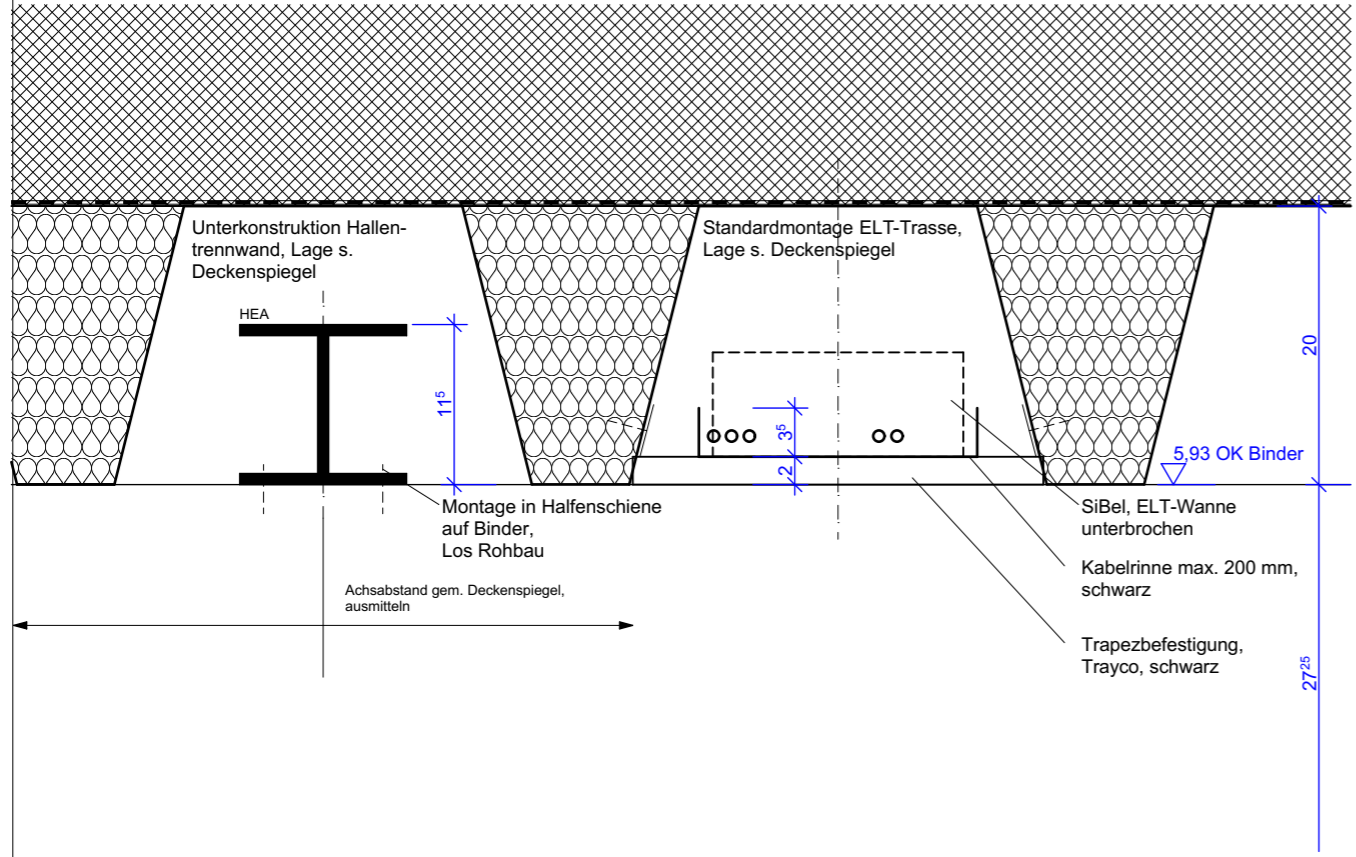
Vertikalschnitt
