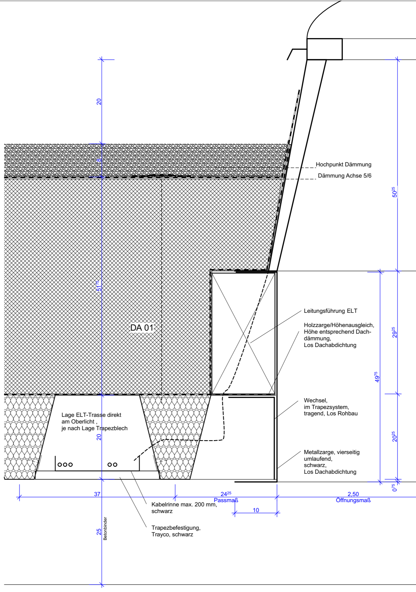
Vertikalschnitt Lichtkuppel
