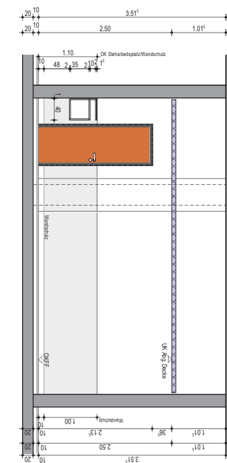
Wandansicht B
