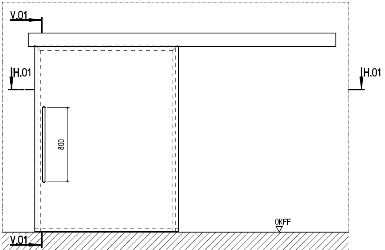
▲ Schematische Tür-Ansicht Antriebsseite
