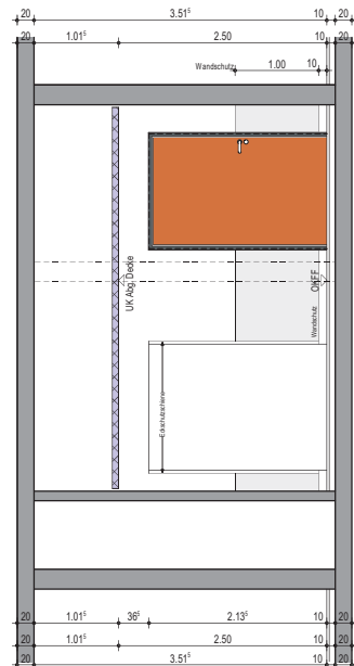
Wandansicht D.1
