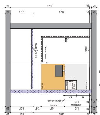
Wandansicht D.1
