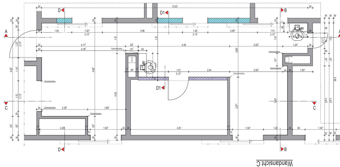
Wandansicht A
