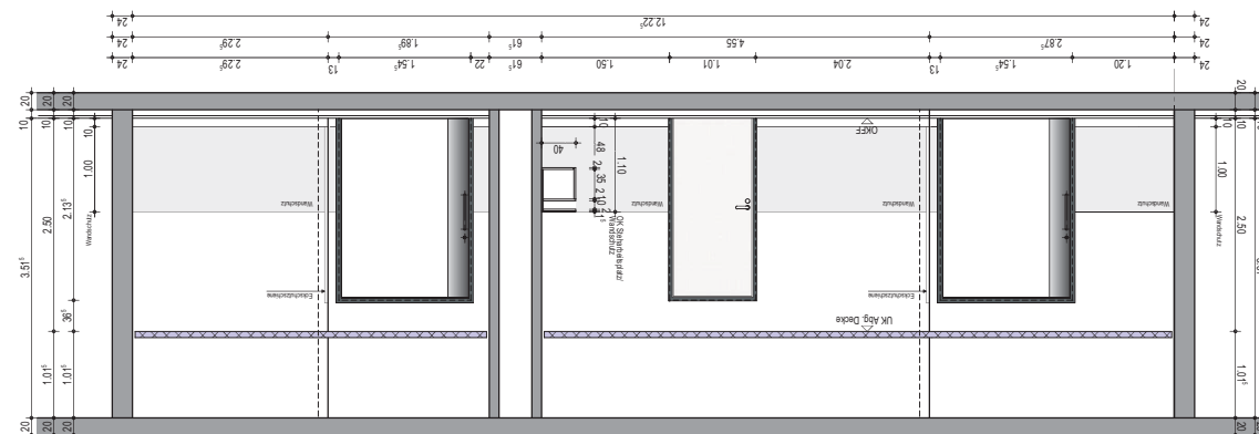
Wandansicht C
